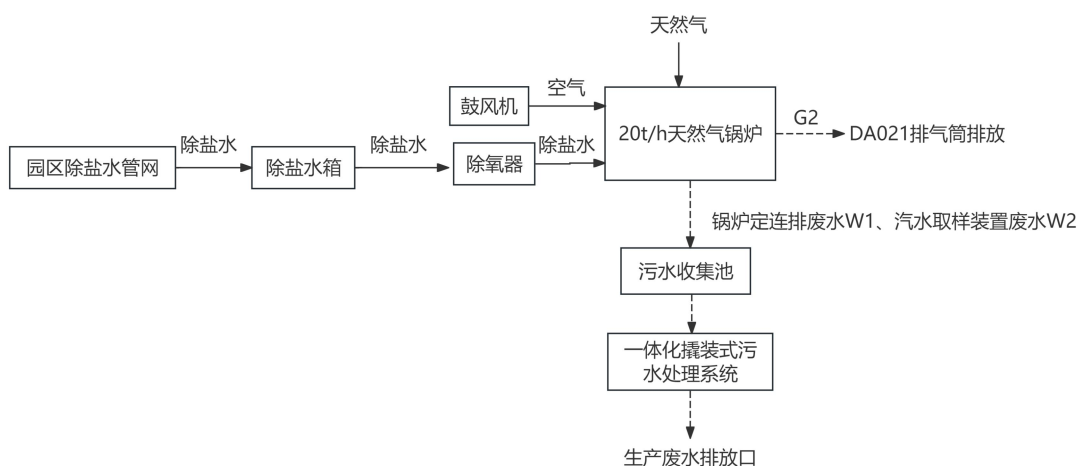
图 2.10-2 天然气锅炉工艺流程及产污环节图
