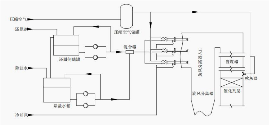
图 5.1-2 典型循环流化床锅炉 SNCR/SCR 联合脱硝工艺流程
