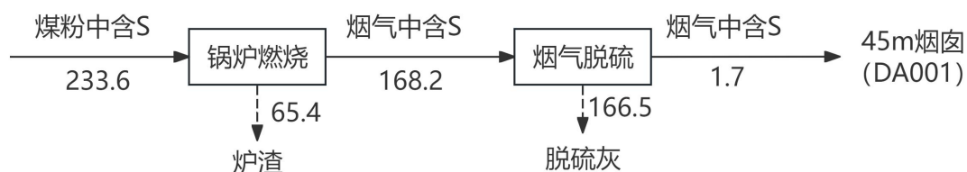
图 2.7-1 本项目设计煤种 S 元素平衡图 (单位: t/a)
