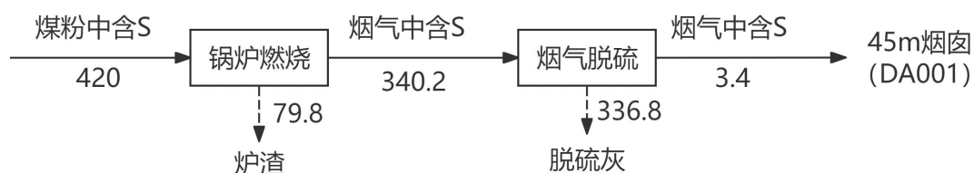
图 2.7-2 本项目校核煤种 S 元素平衡图 (单位: t/a)
