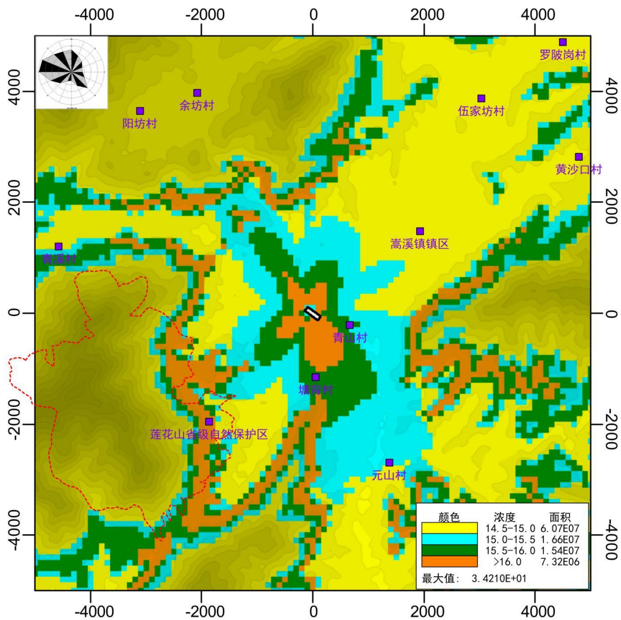
图 4.8-7 叠加后 NO 2 区域保证率下 24 小时平均浓度网格分布图(单位: µg/m 3 )
