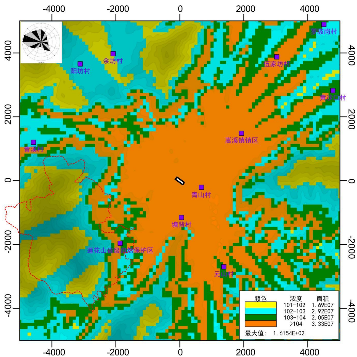
图 4.8-9 叠加后氨区域 1 小时平均浓度网格分布图(单位: \mu\text{g}/\text{m}^3 )
