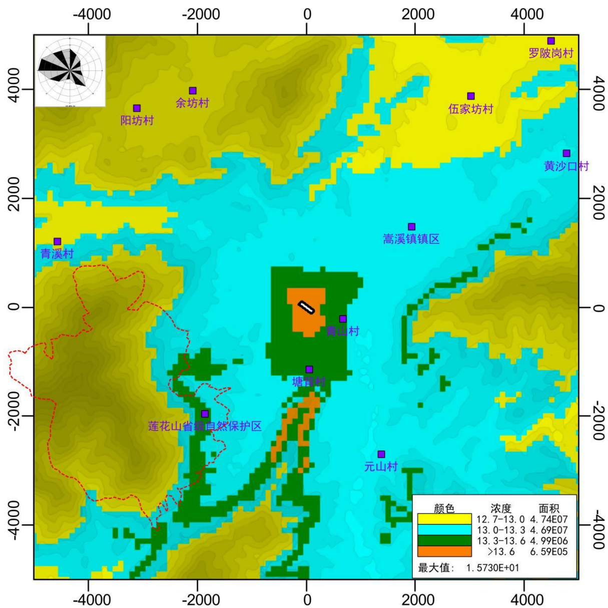
图 4.8-4 叠加后 PM 2.5 区域年平均浓度网格分布图(单位: \mu\text{g}/\text{m}^3 )
