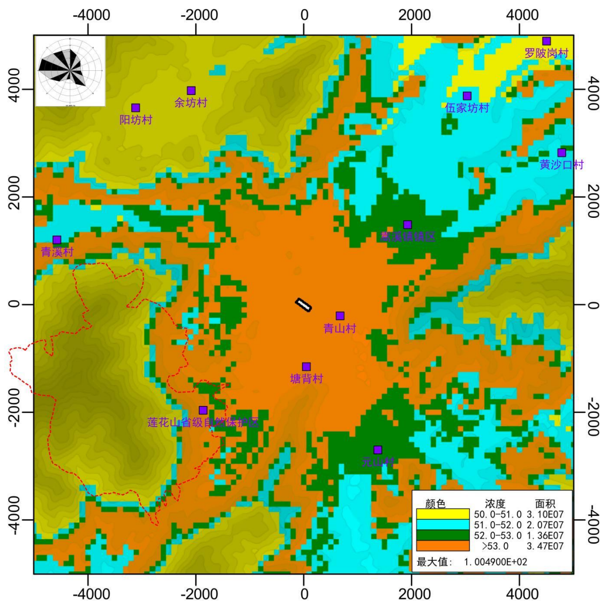
图 4.8-1 叠加后 PM_{10} 区域保证率下 24 小时平均浓度网格分布图(单位: \mu g/m^3 )
