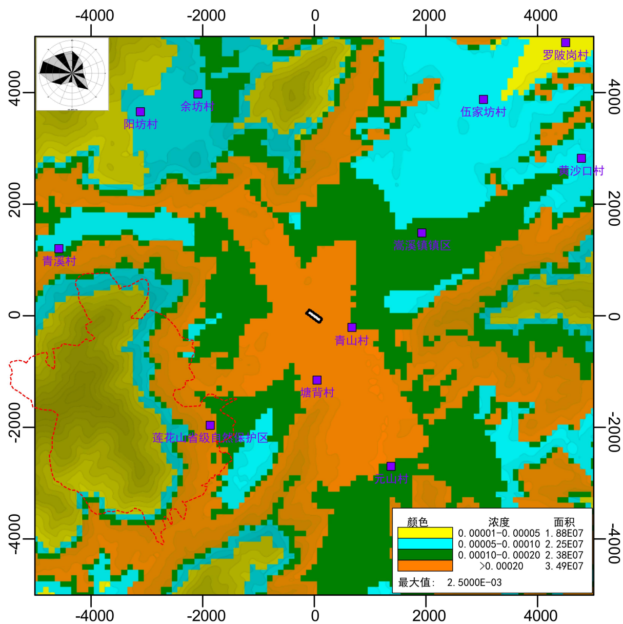
图 4.8-11 叠加后汞区域 24 小时平均浓度网格分布图(单位: \mu\text{g}/\text{m}^3 )
