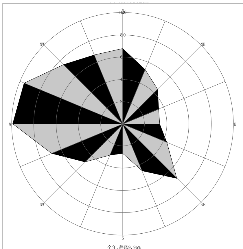
图 4.1-1 清流县全年风向玫瑰图（静风频率 9.95%）
