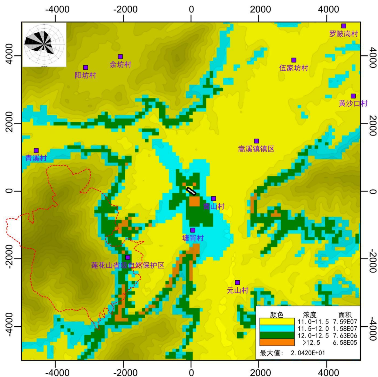
图 4.8-5 叠加后 SO 2 区域保证率下 24 小时平均浓度网格分布图(单位: \mu\text{g}/\text{m}^3 )
