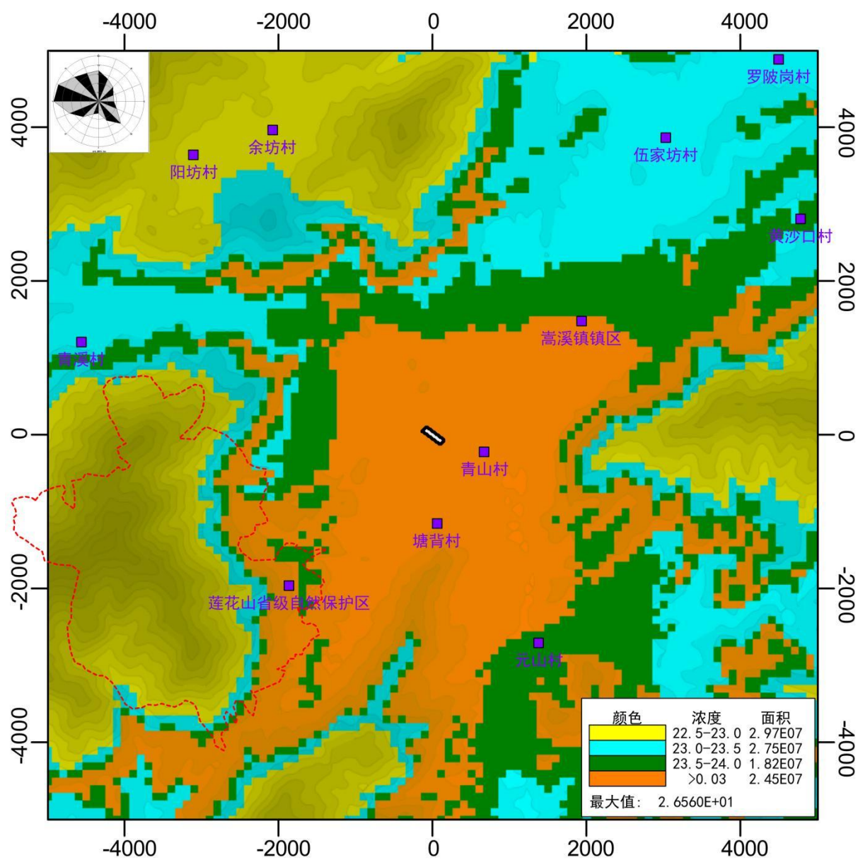
图 4.8-2 叠加后 PM 10 区域年平均浓度网格分布图(单位: \mu\text{g}/\text{m}^3 )
