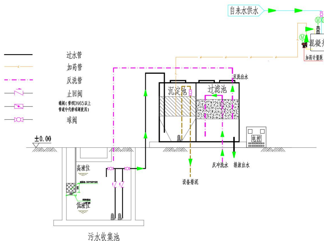
图 4.2-1 污水处理工艺流程图
