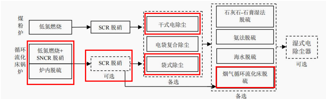
图5.1-1 超低排放技术路线
