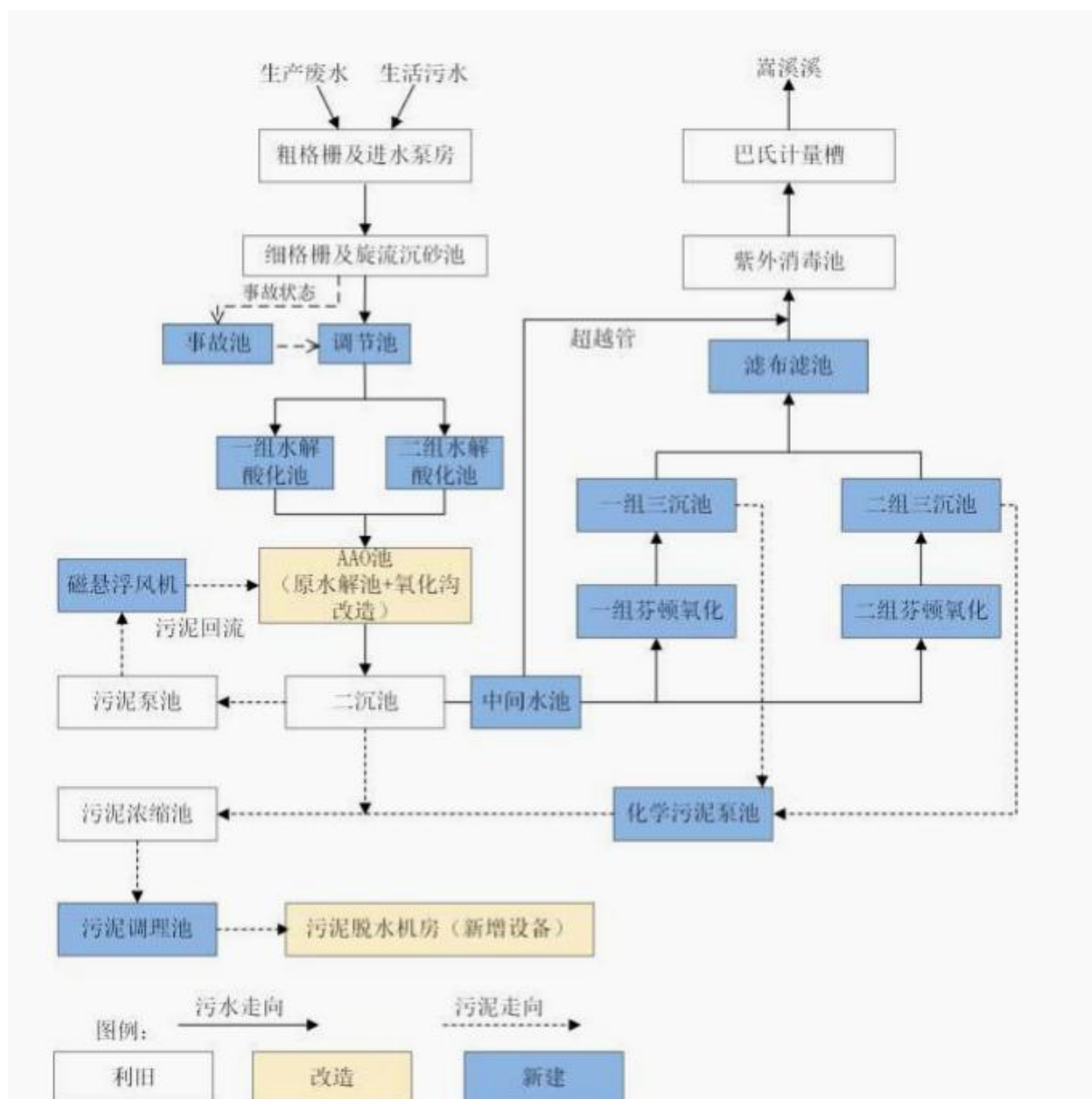
图 4.2-2 嵩溪镇污水处理厂污水处理工艺流程图
