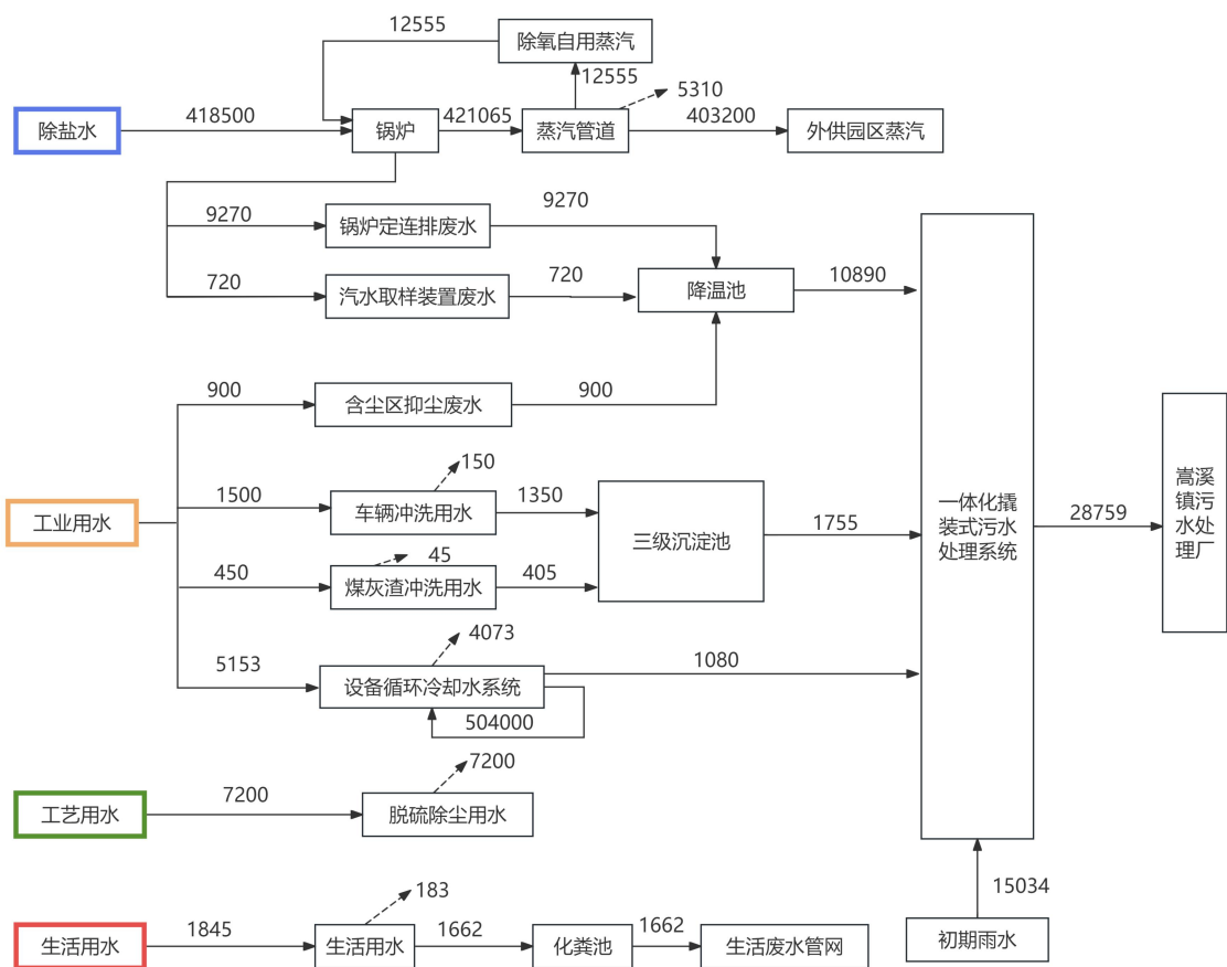
图2.6-1 本项目水平衡图（单位：m³/a）
