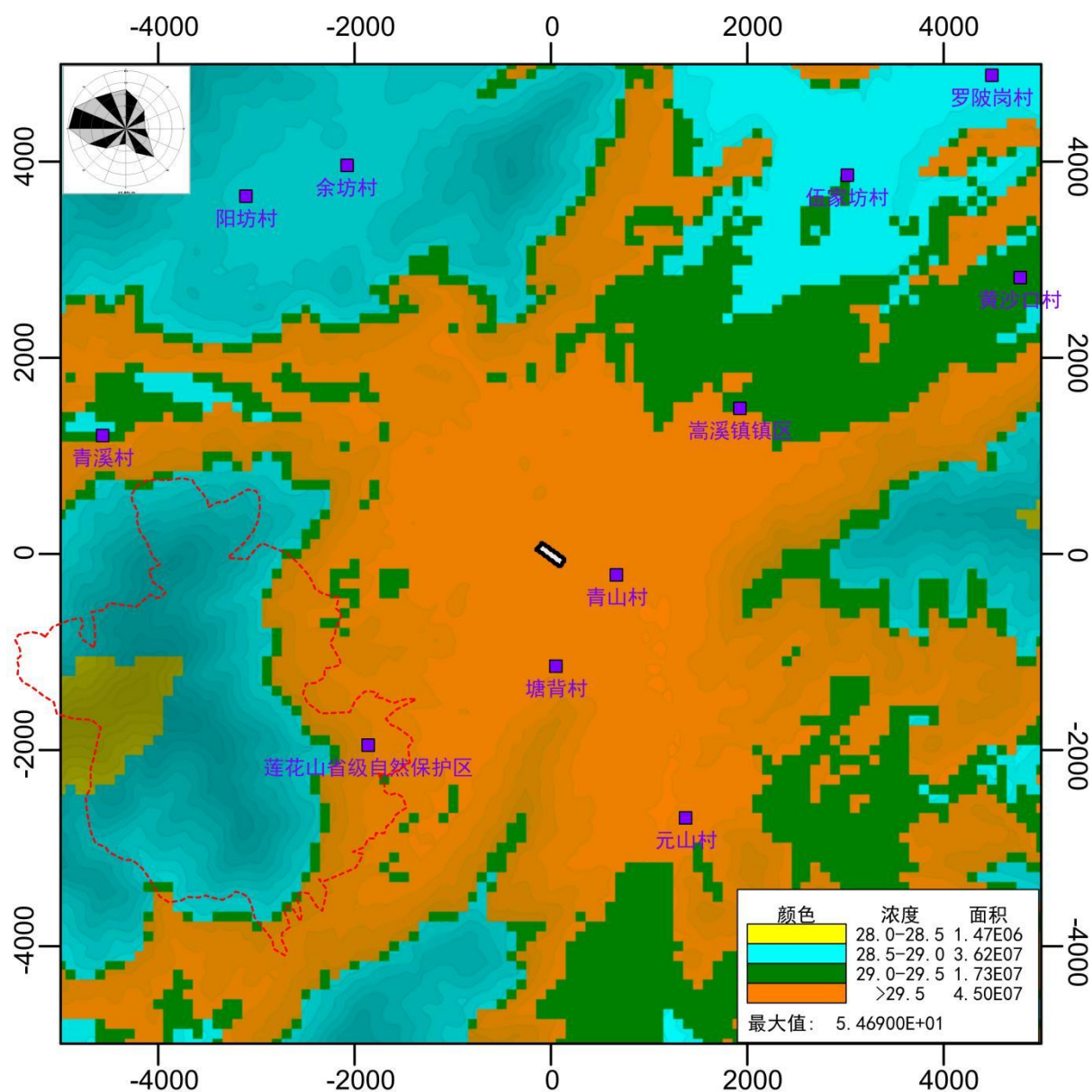
图 4.8-3 叠加后 PM 2.5 区域保证率下 24 小时平均浓度网格分布图(单位: \mu\text{g}/\text{m}^3 )
