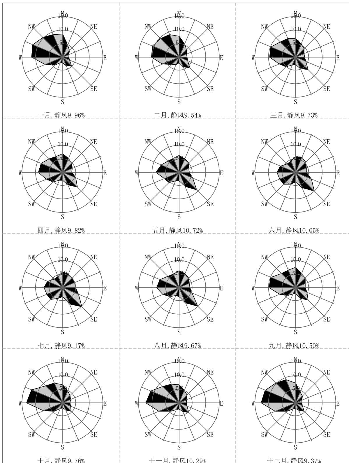
图 4.1-2 清流县月风向玫瑰图
