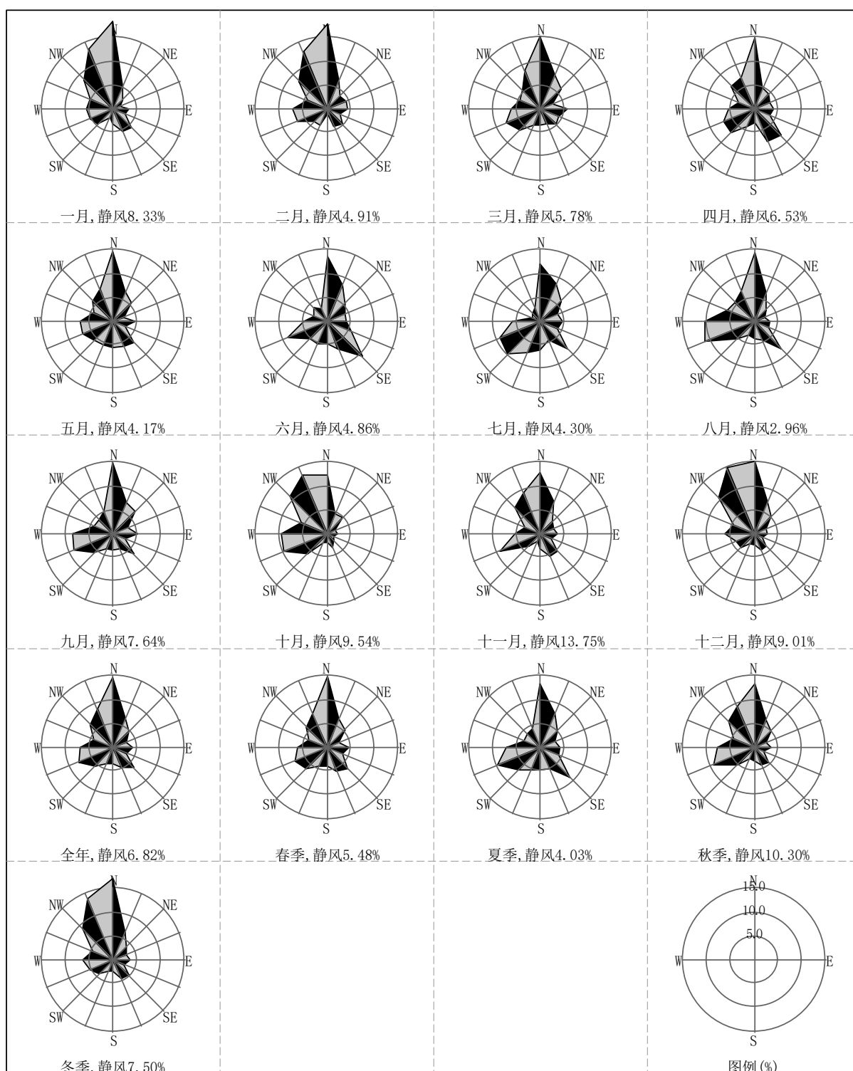
图 4.1-6 清流县 2023 年风向风频玫瑰图
