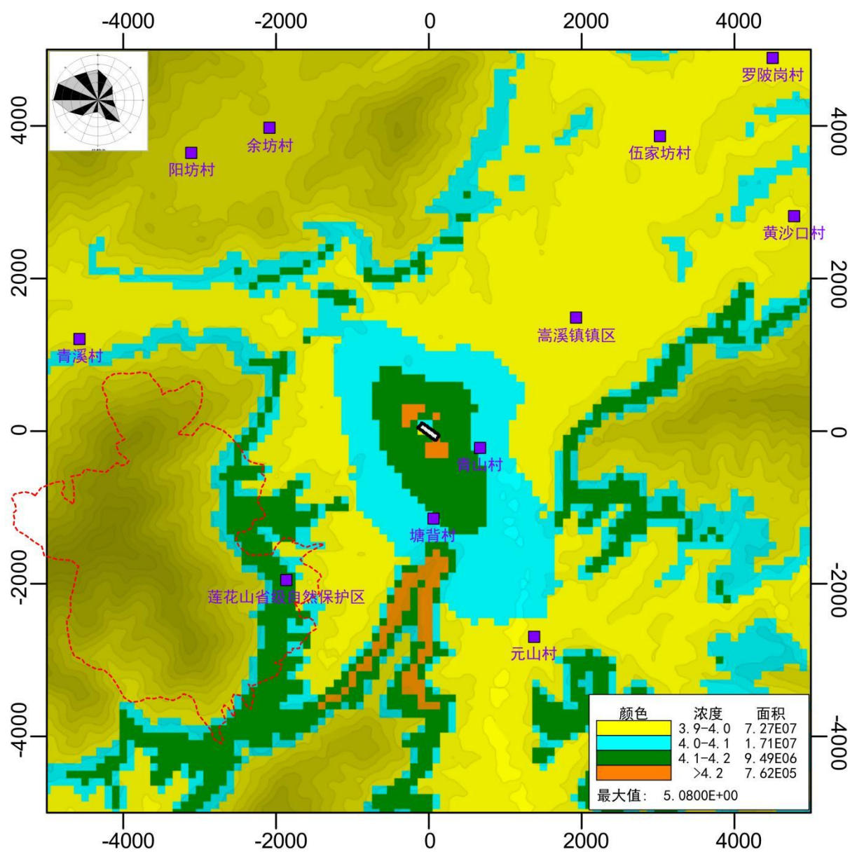
图 4.9-6 叠加后 SO 2 区域年平均浓度网格分布图(单位: \mu\text{g}/\text{m}^3 )
