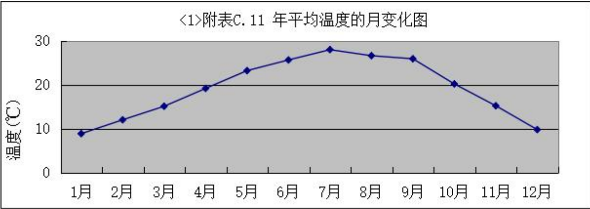
图 4.1-3 年平均温度变化曲线
