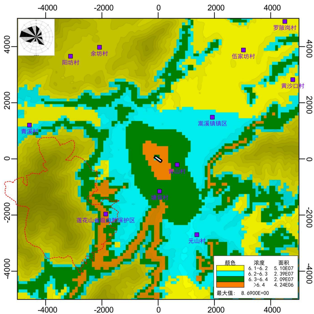
图 4.8-8 叠加后 NO 2 区域年平均浓度网格分布图(单位: \mu\text{g}/\text{m}^3 )
