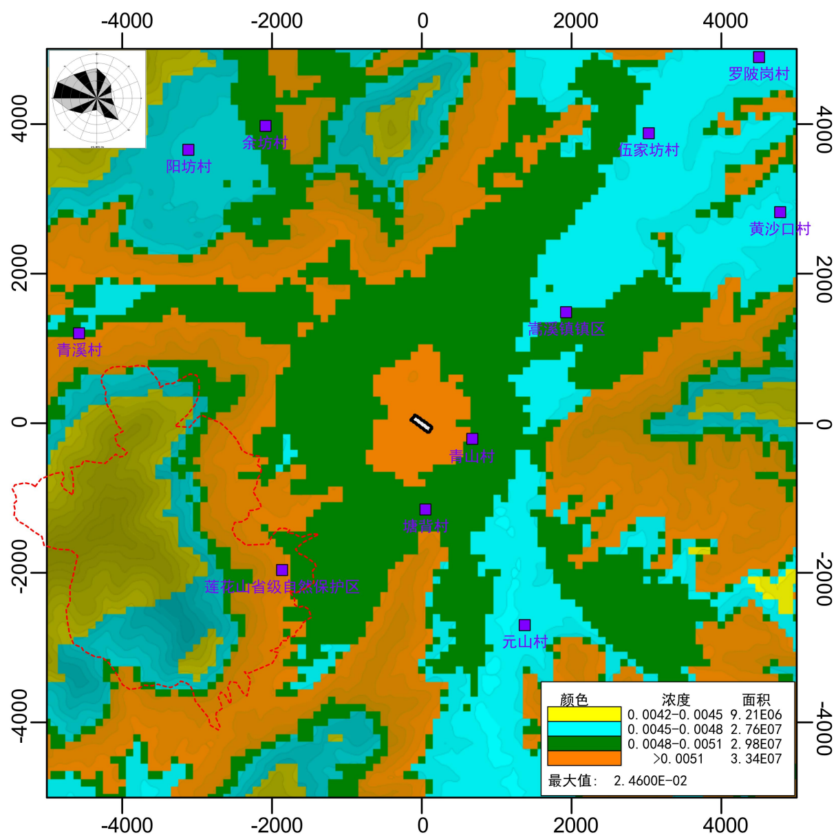
图 4.8-10 叠加后汞区域 1 小时平均浓度网格分布图(单位: \mu\text{g}/\text{m}^3 )
