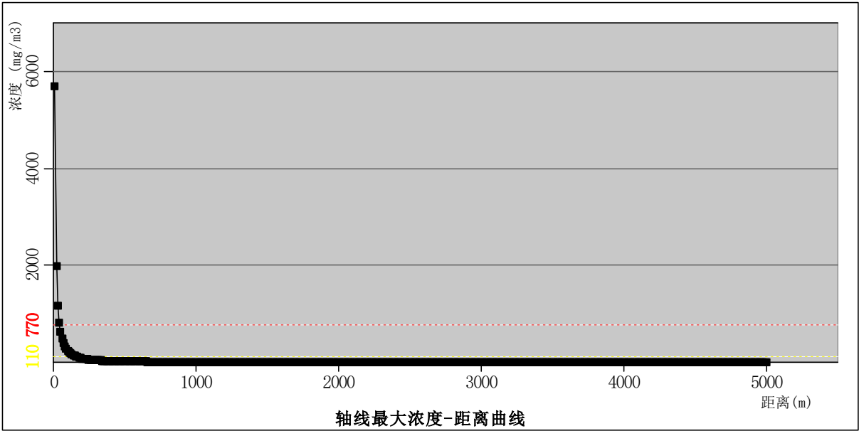
图 5.1-1 氨水储罐泄漏轴线最大浓度距离曲线（最不利气象条件）
