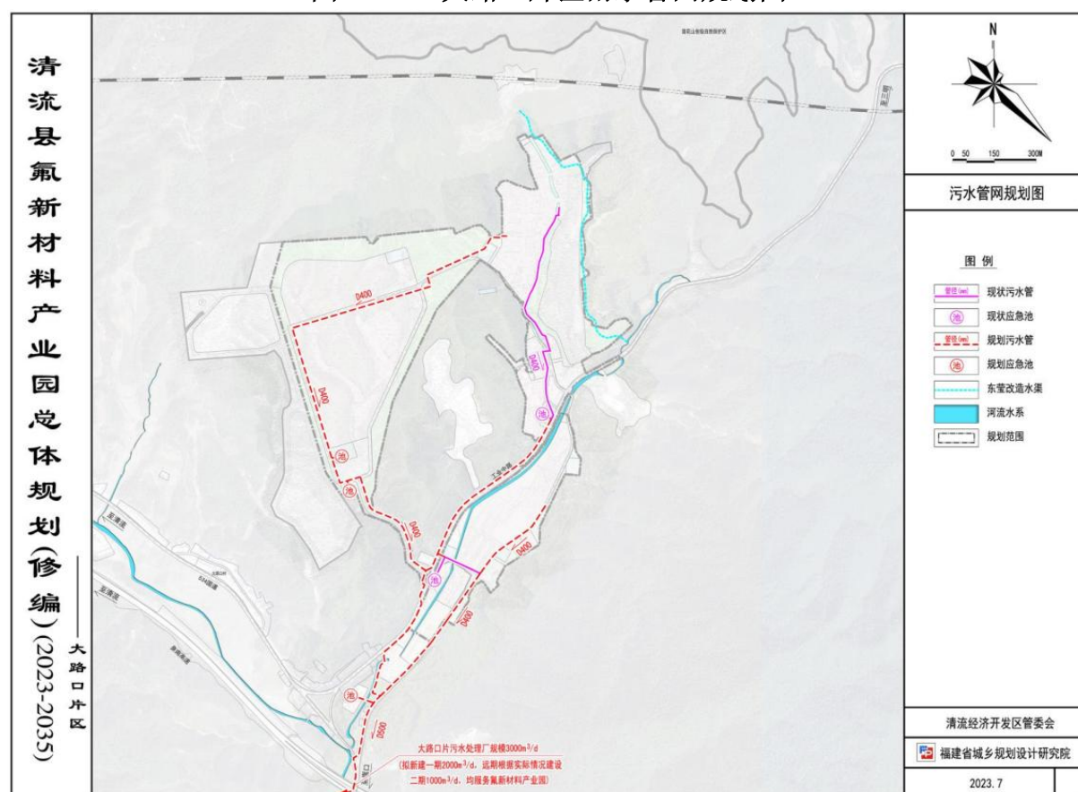
图 1.7-6 大路口片区污水管网规划图
