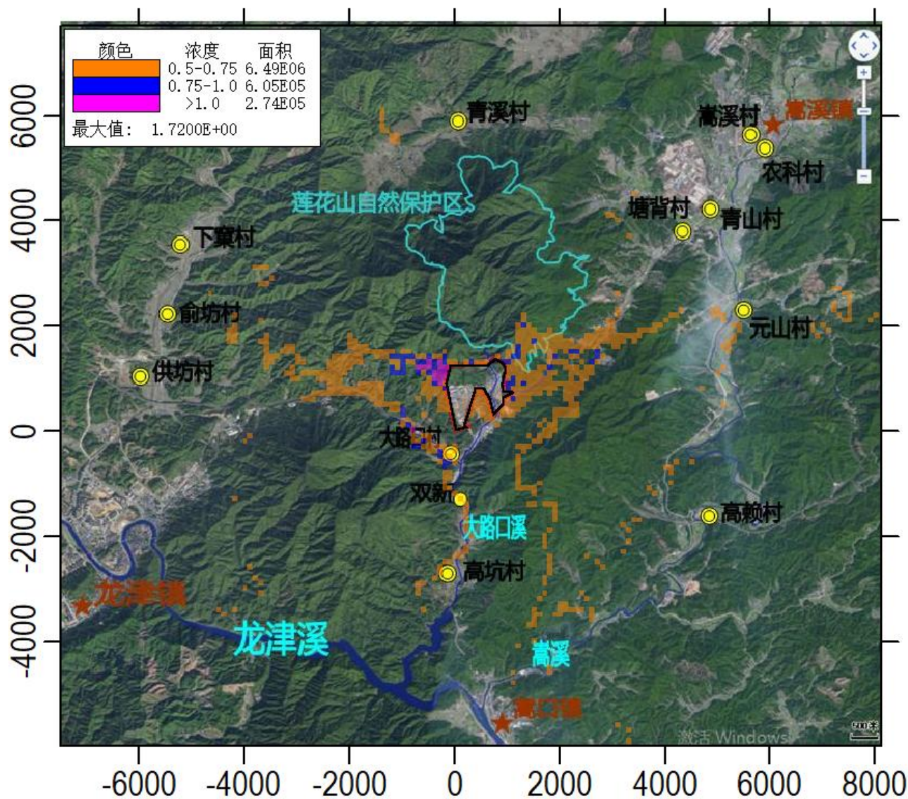
图 5.1-6 氟化物最大落地日平均浓度分布图 单位: \mu\text{g}/\text{m}^3
