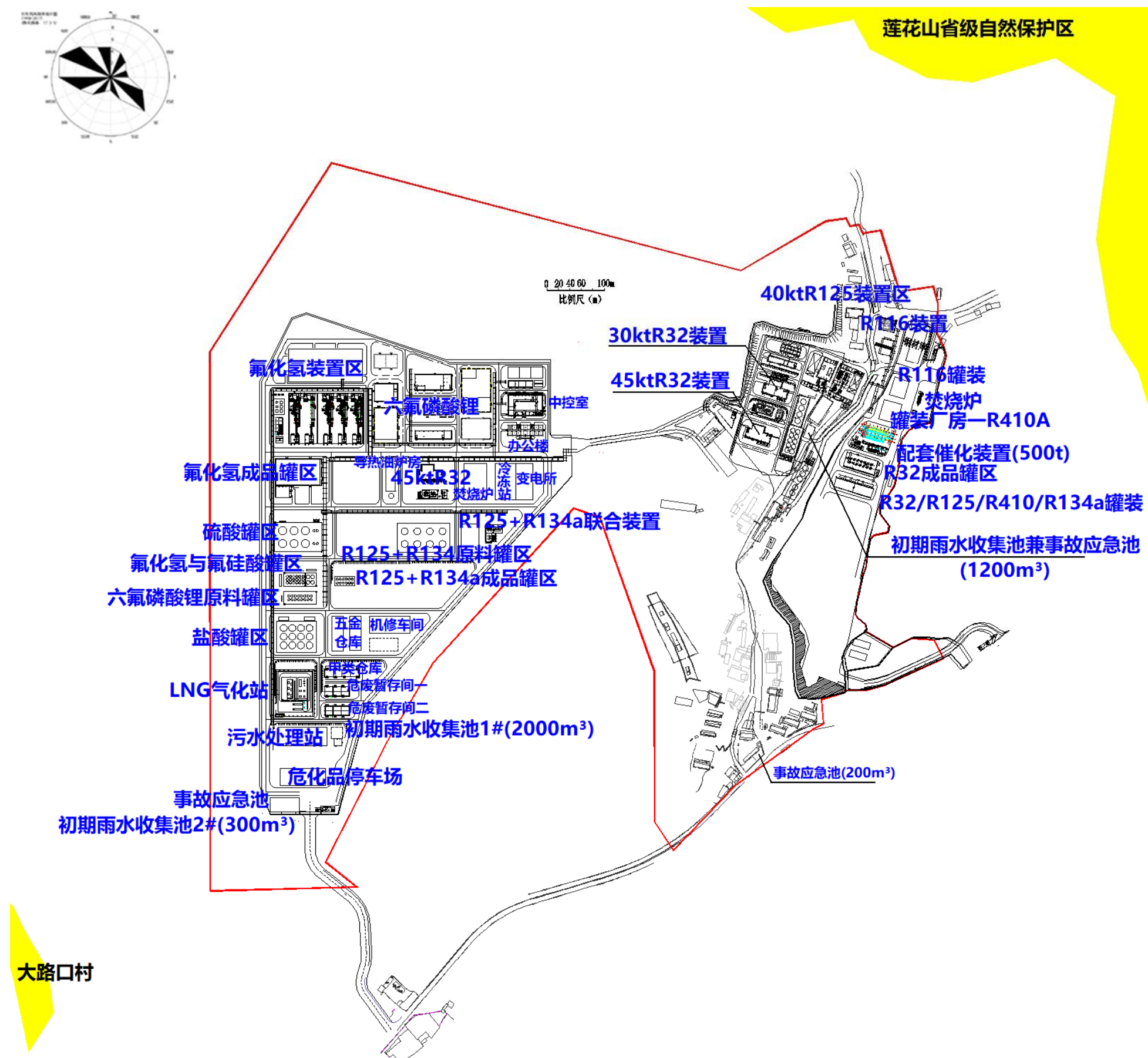
图 2.3-4 现有已建+在建+以新带老工程实施后全厂总平布局图
