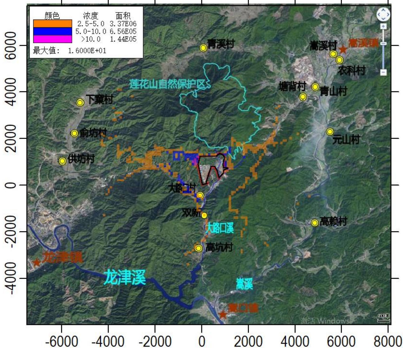
图 5.1-5 氟化物最大落地小时平均浓度分布图 单位: \mu\text{g}/\text{m}^3
