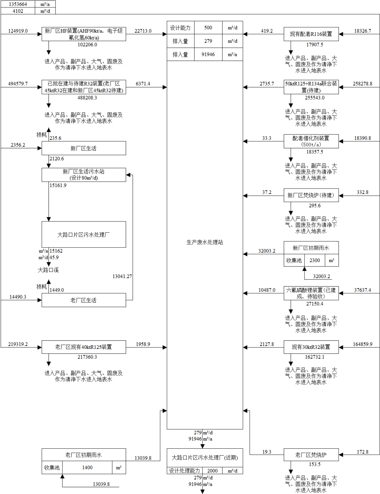
图 3.5-6 本次改建后全厂水平衡图
