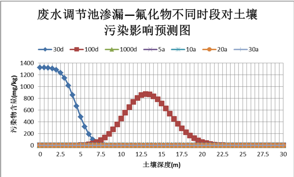
图 5.5-2 废水调节池渗漏——氟化物对不同时段对土壤污染影响预测图
