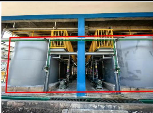
AHF 车间综合废气处理设施(3 级氢氧化钙除氟, 一用一备)
