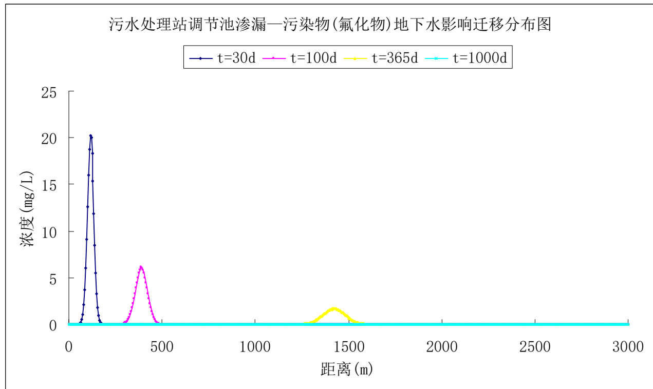
图 5.4-3 污水处理站调节池渗漏情景污染物-氟化物地下水迁移图
