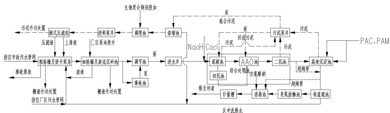
图 5.3-1 大路口片区新污水处理厂工艺流程图
