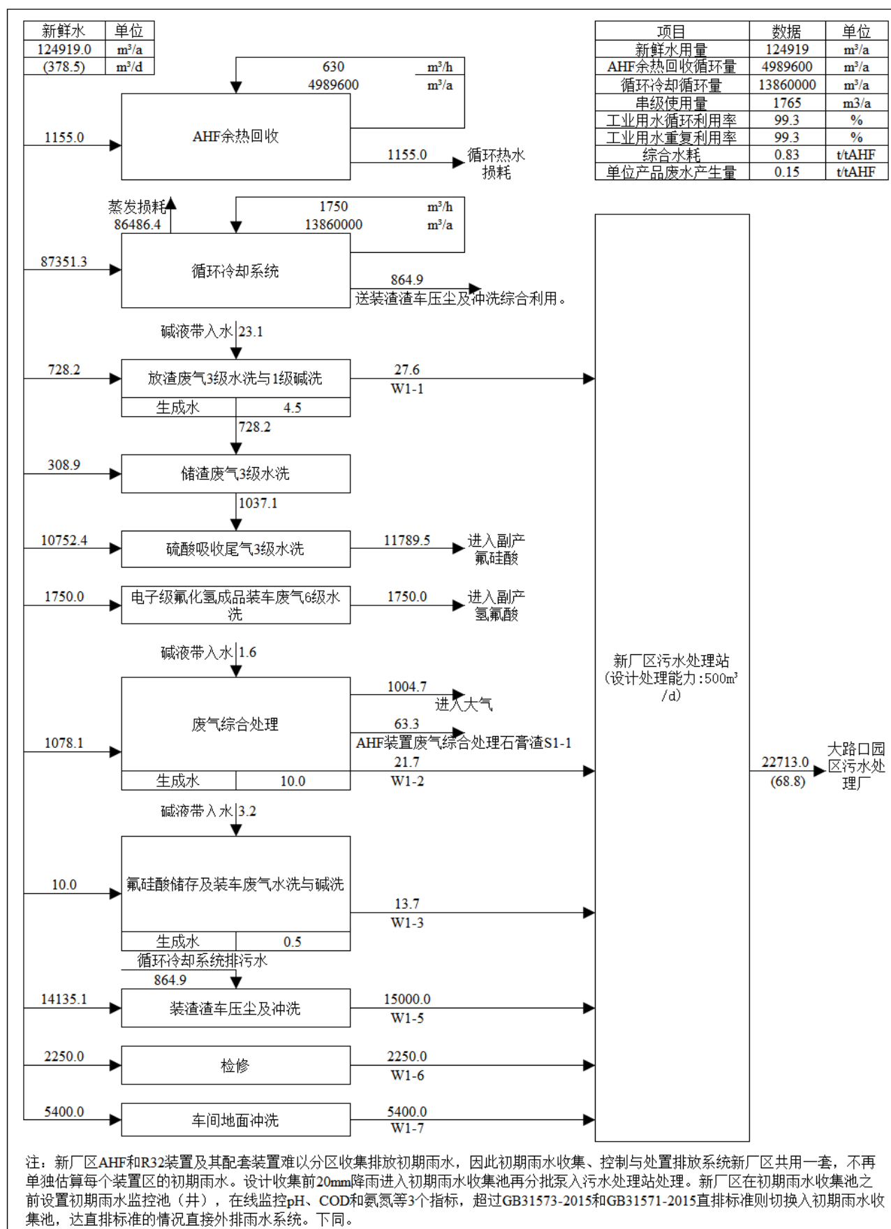
图 3.5-5 本次改建后新厂区氟化氢装置(AHF9 万吨/年+电子级氟化氢 6 万吨/年)水平衡图
