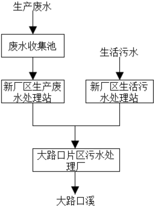
图 2.5-3 企业现有废水收集与处理系统图
