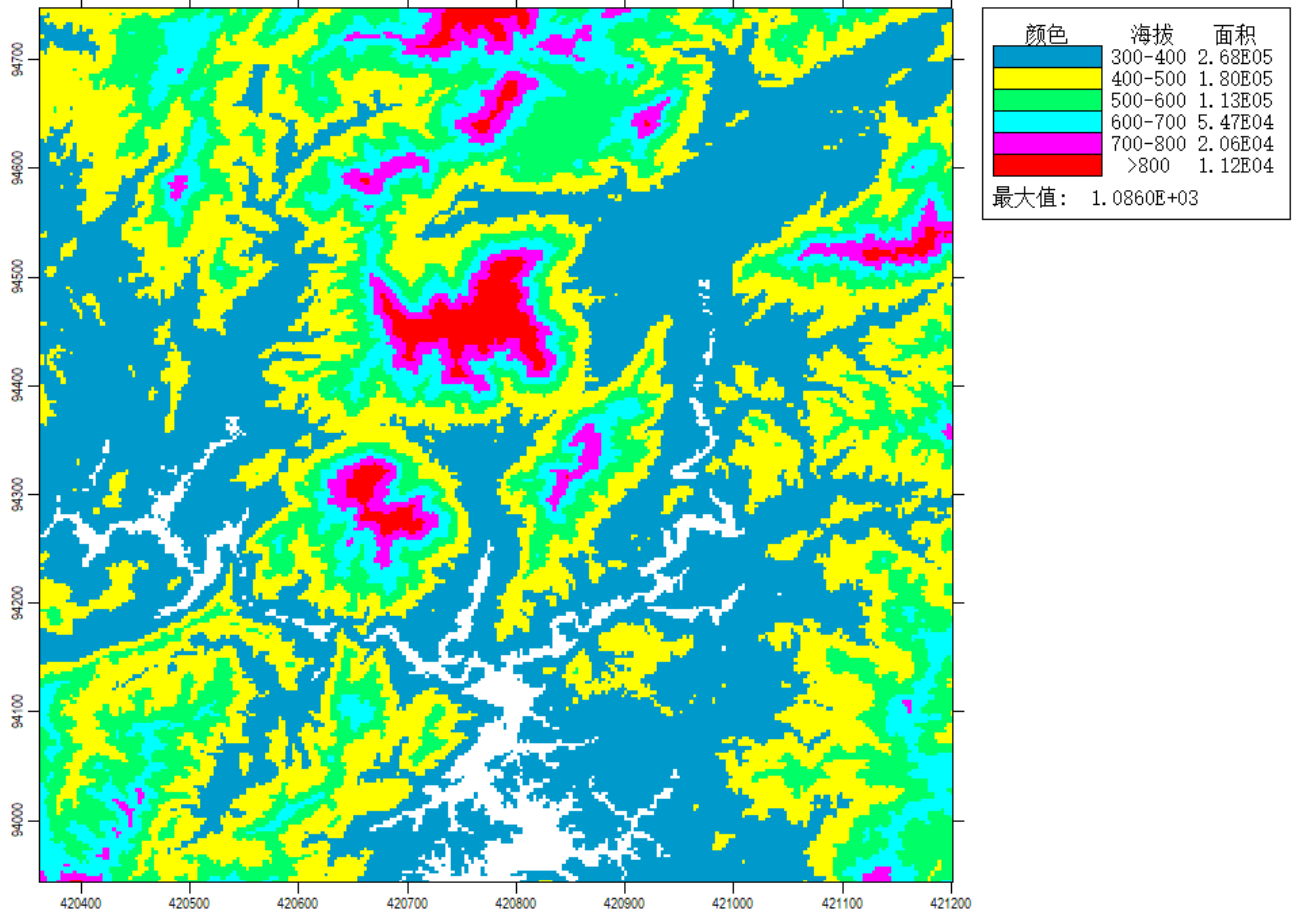
图 5.1-2 地形高程图
