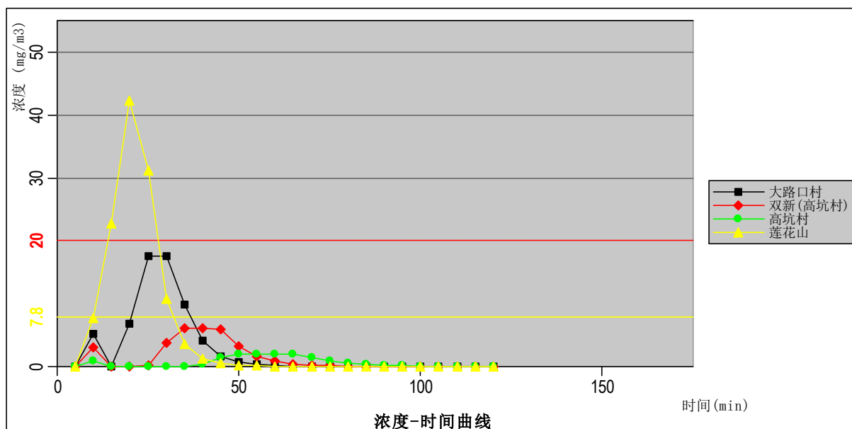
图 6.6-10 最常见气象条件下氟氮气瓶泄漏-各关心点氟气浓度-时间变化图
