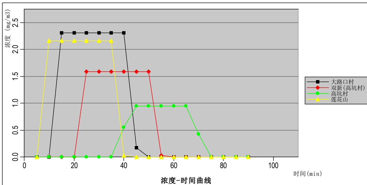
图 6.6-2 最不利气象条件下氟化氢泄漏-各关心点氟化氢浓度-时间变化图
