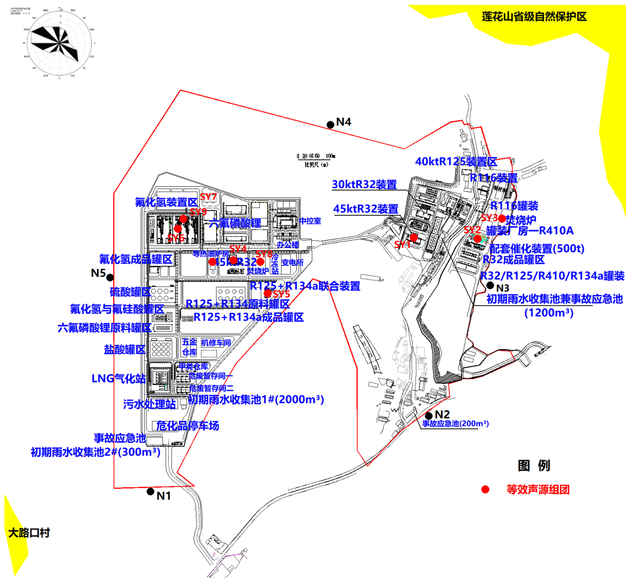
图 5.7-1 本次评价声环境影响预测相关等效声源组团分布图
