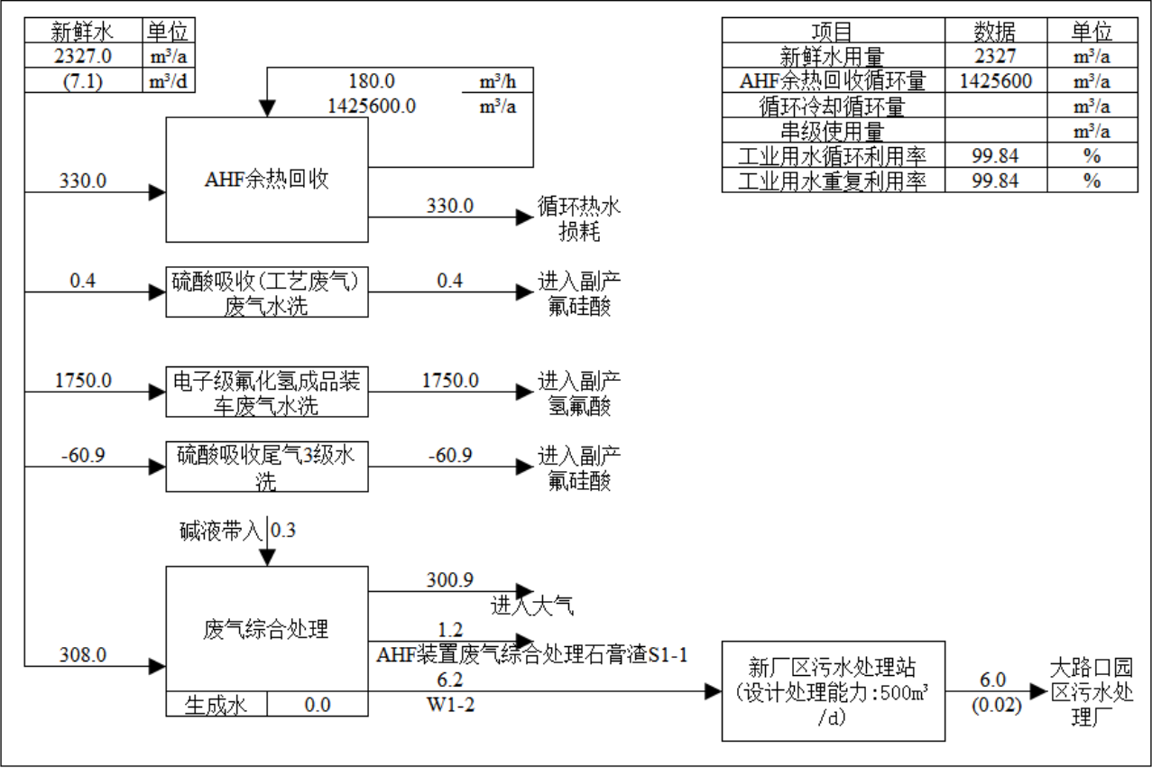
图 3.5-4 本次改建工程水平衡图
