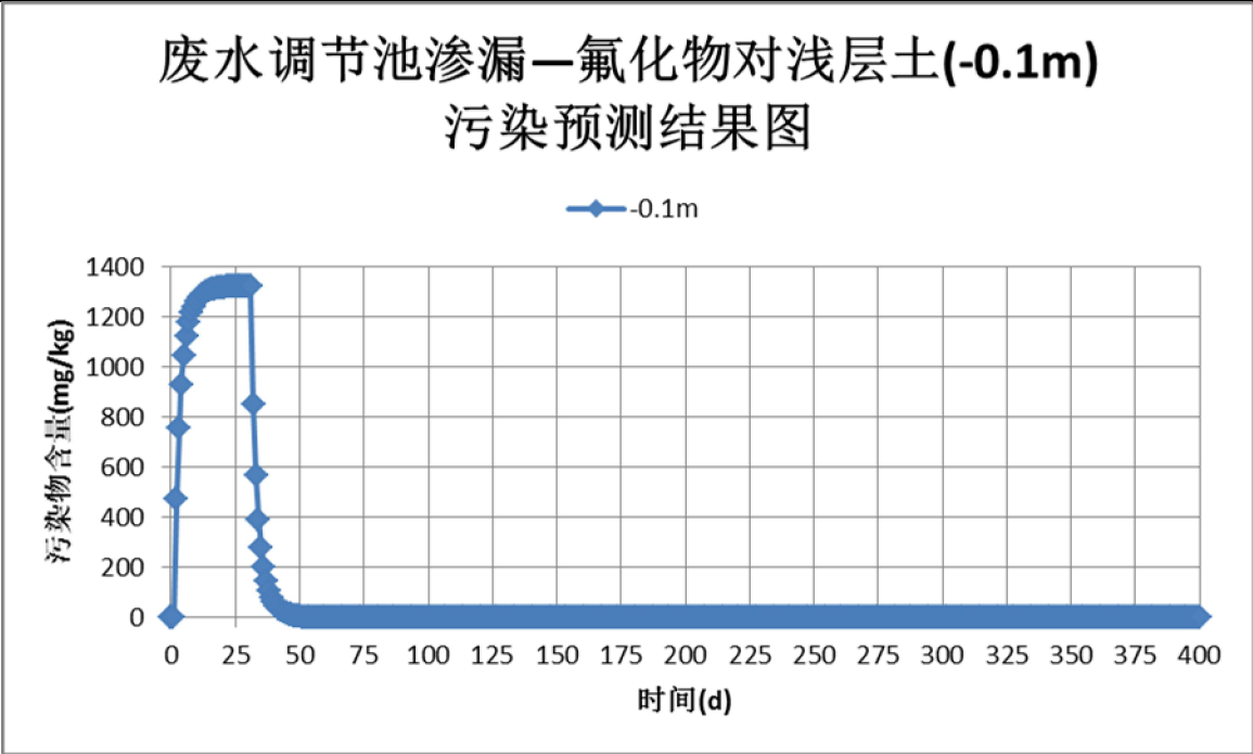
图 5.5-1 废水调节池渗漏——氟化物对浅层土壤污染预测结果图
