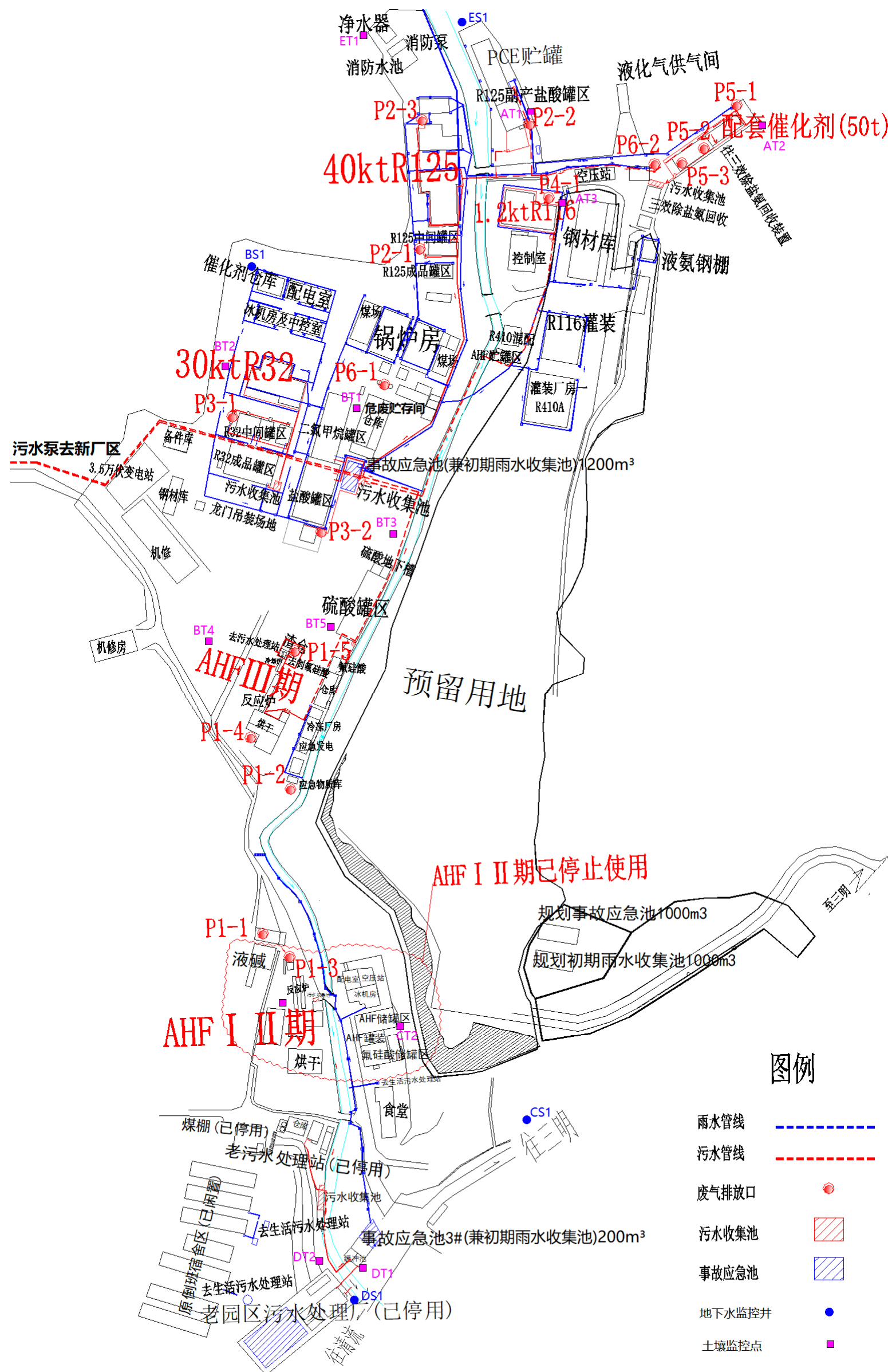
图 2.3-1 老厂区已建工程总平布局、雨污管网及主要环保设施分布图
