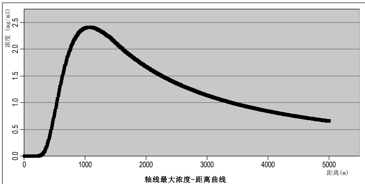
图 6.6-1 最不利气象条件下氟化氢泄漏-下风向轴线最大浓度图
