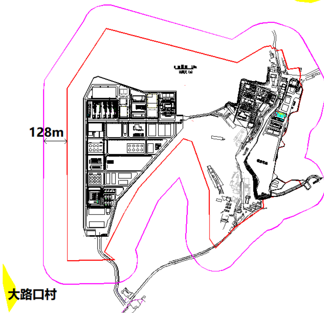
图 5.1-7 本次改建后企业环境防护距离包络图
