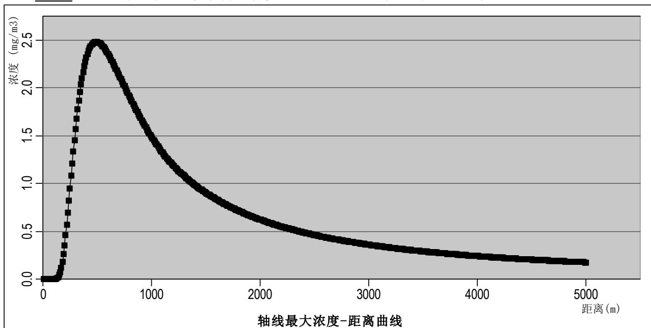
图 6.6-3 最常见气象条件下氟化氢泄漏-下风向轴线最大浓度图
