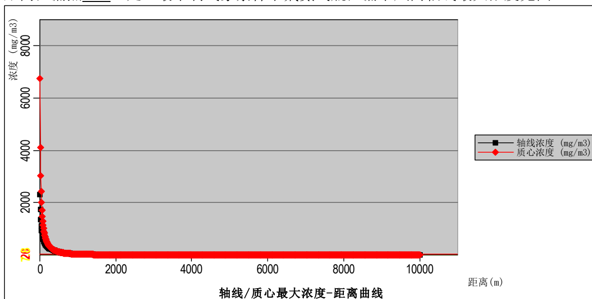
图 6.6-5 最不利气象条件下氟氮气瓶泄漏-下风向轴线最大浓度图
