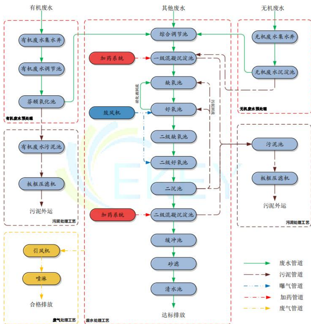
图 2.5-5 现有生产废水处理工艺流程图
