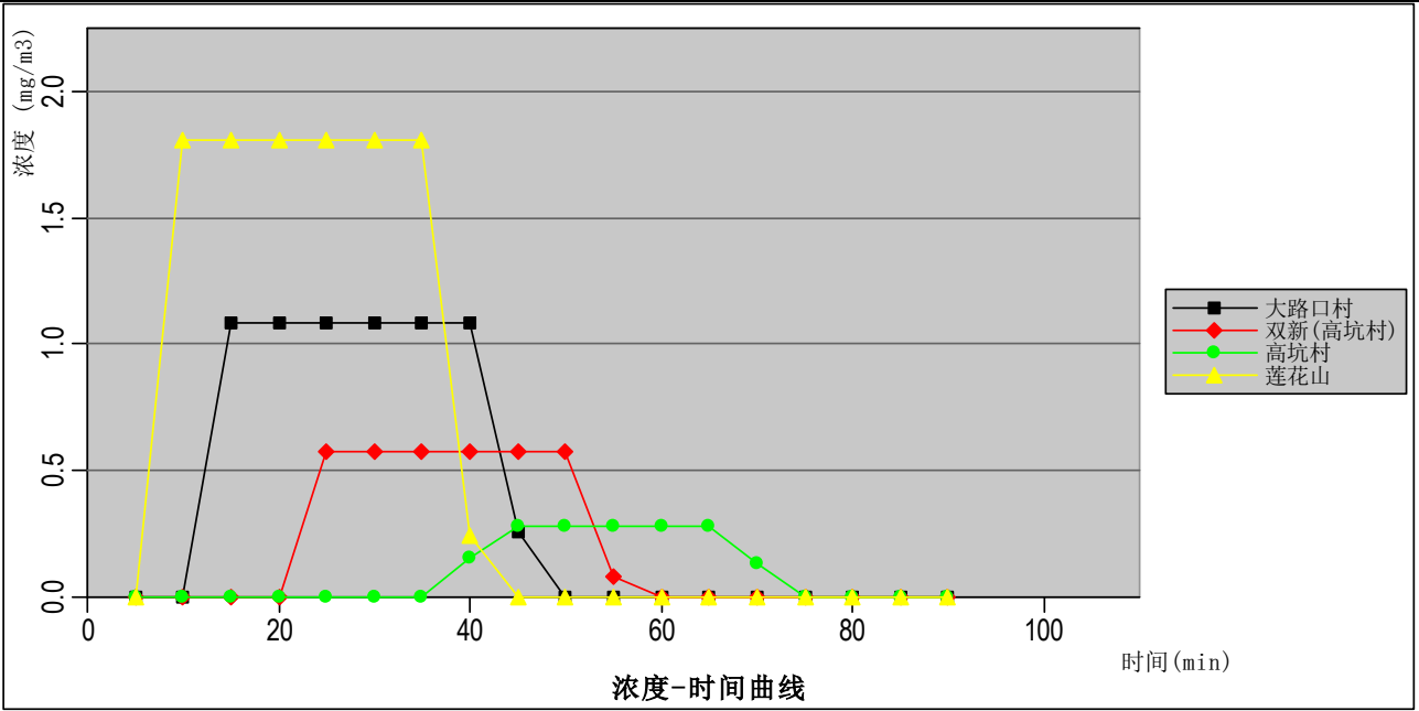
图 6.6-4 最常见气象条件下氟化氢泄漏-各关心点氟化氢浓度-时间变化图
