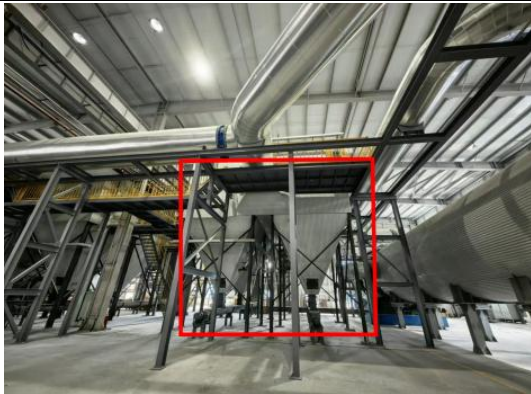
萤石烘干废气、储粉粉尘预处理设施[布袋除尘(含重力除尘)]
