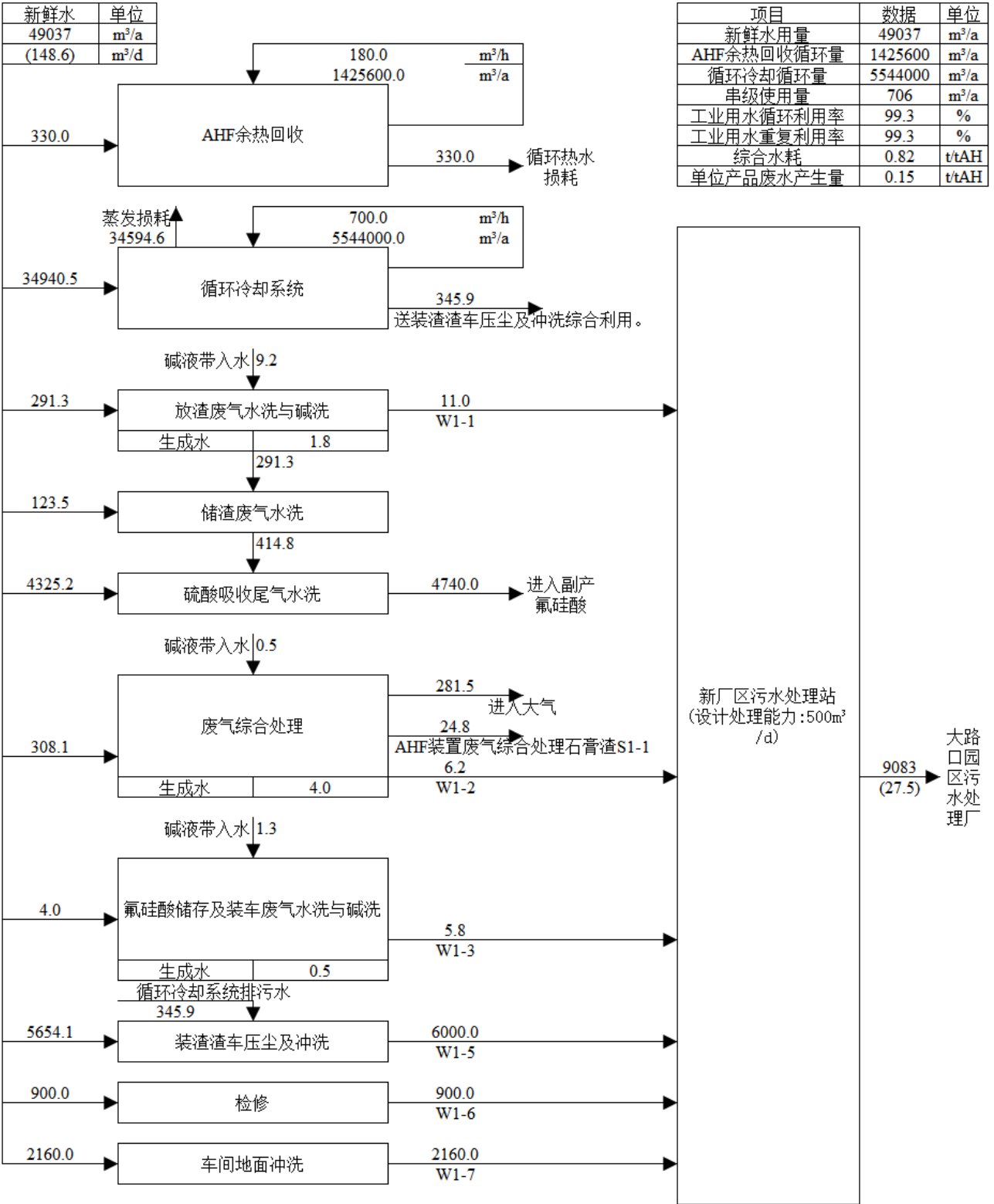
图 2.5-8 新厂区现有已建 60KtAHF 装置水平衡图
