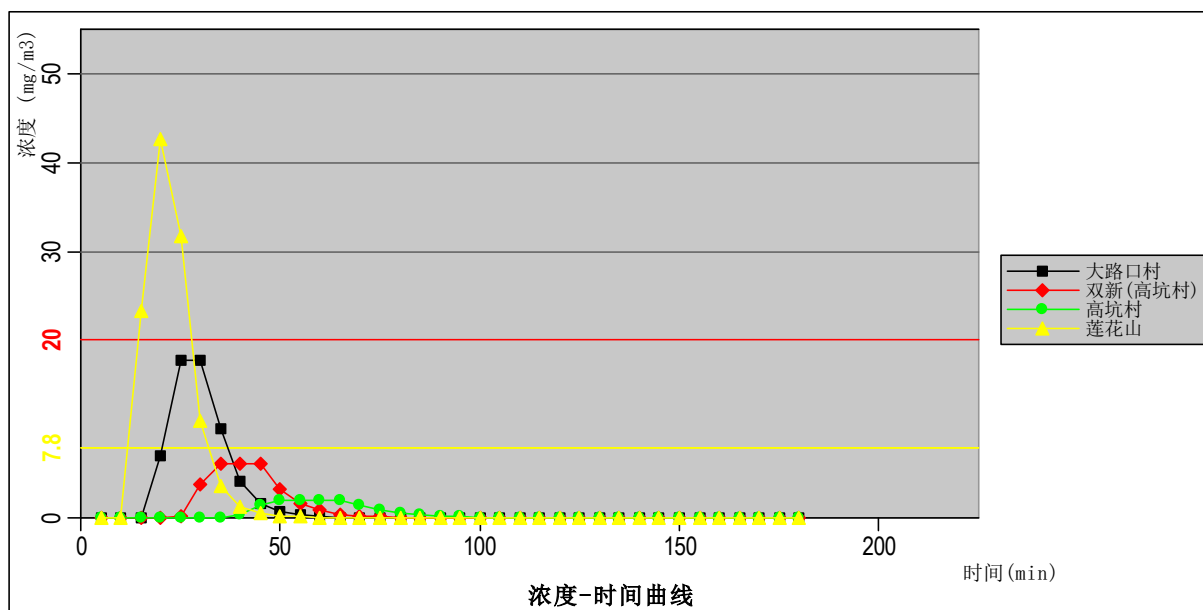
图 6.6-7 最不利气象条件下氟氮气瓶泄漏-各关心点氟气浓度-时间变化图
