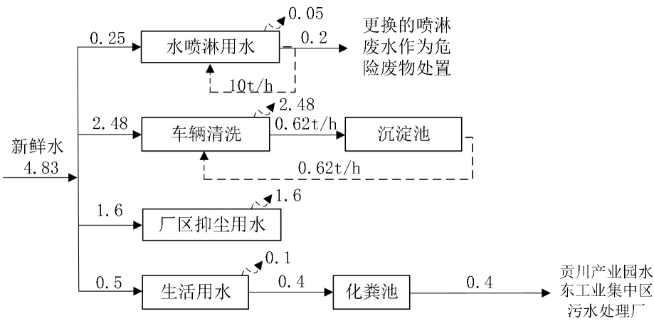
图 2.6-1 项目水平衡单位：t/d
