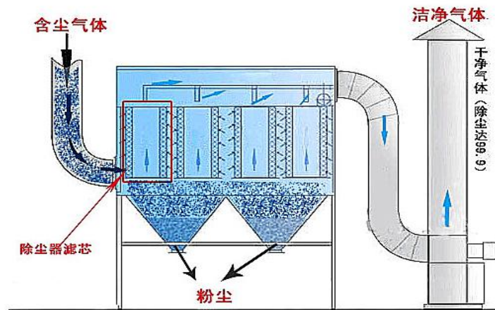
图 7.7-1 布袋除尘装置示意图
