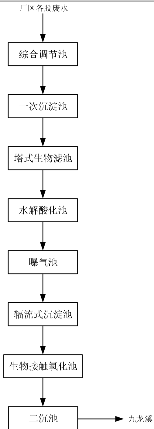
图 2.3-2 废水处理工艺流程图
