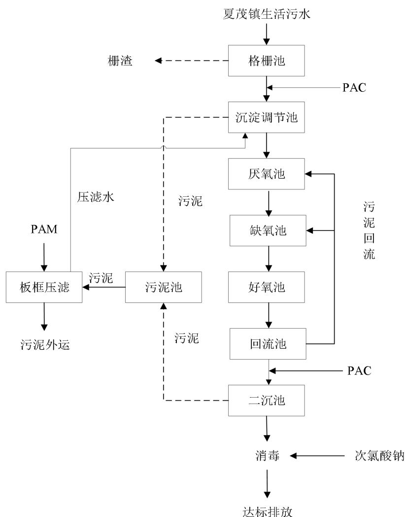
图 5.1-1 项目污水处理工艺流程图
