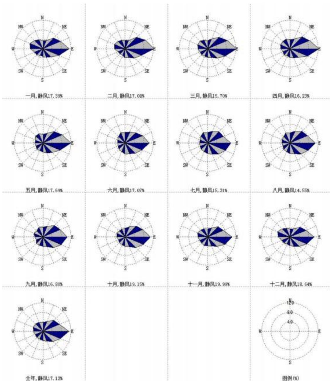
图 4-1 尤溪站 2004~2023 年平均风向频率玫瑰图
