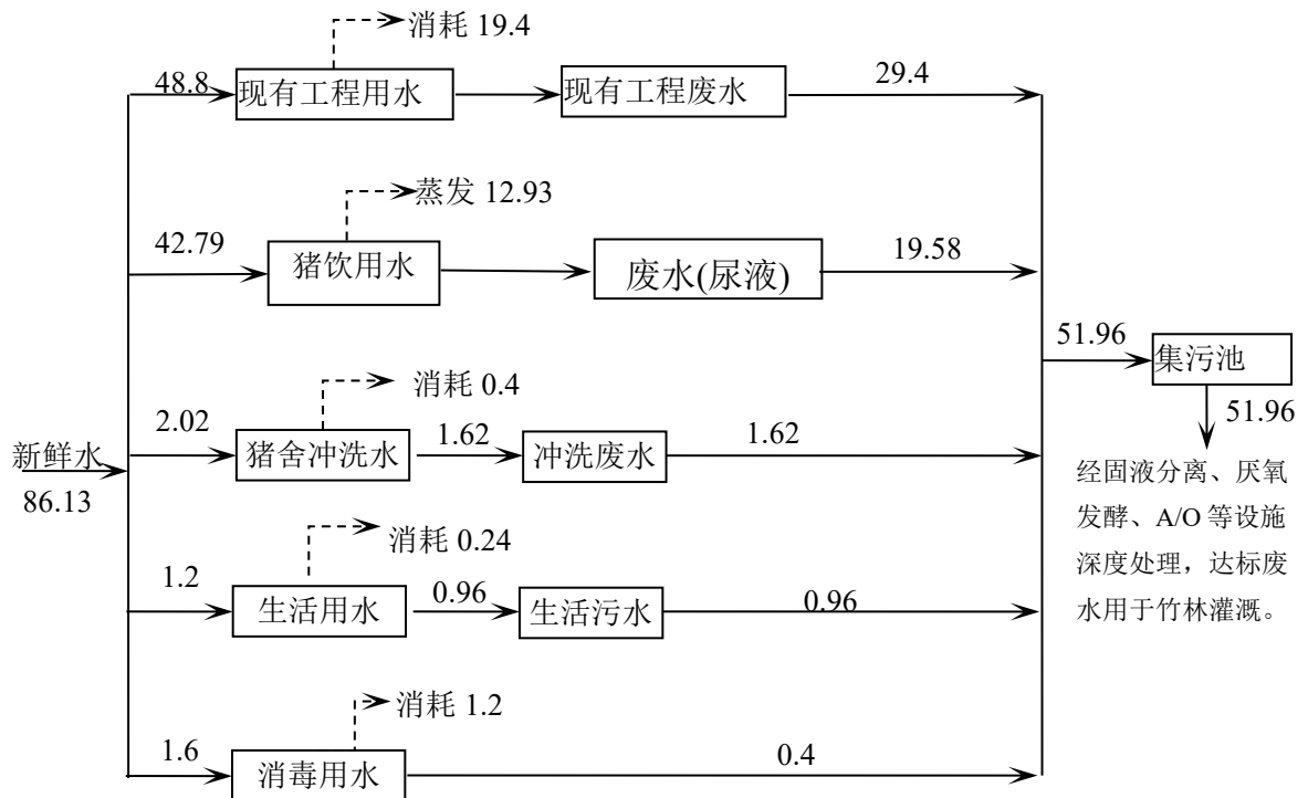
图 2.4-1 春、秋季全场水平衡图（单位 t/d）
