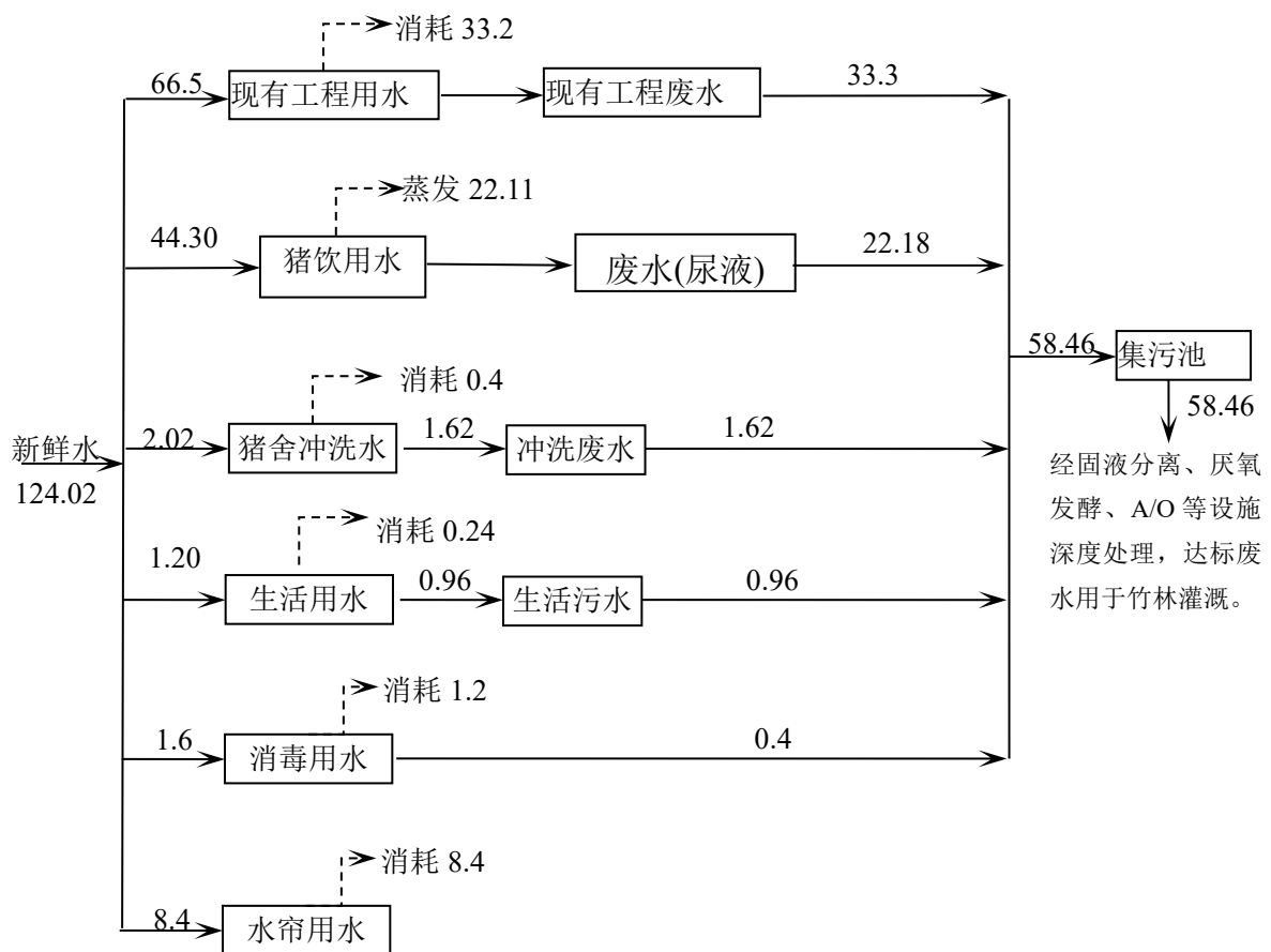
图 2.4-2 夏季全场水平衡图（单位 t/d）
