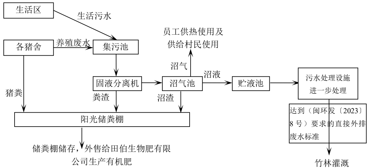
图 2.3-4 项目资源化利用工艺流程
