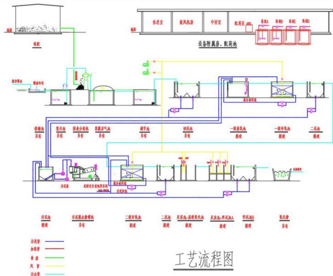
图 5.1-2 污水处理工艺流程图
