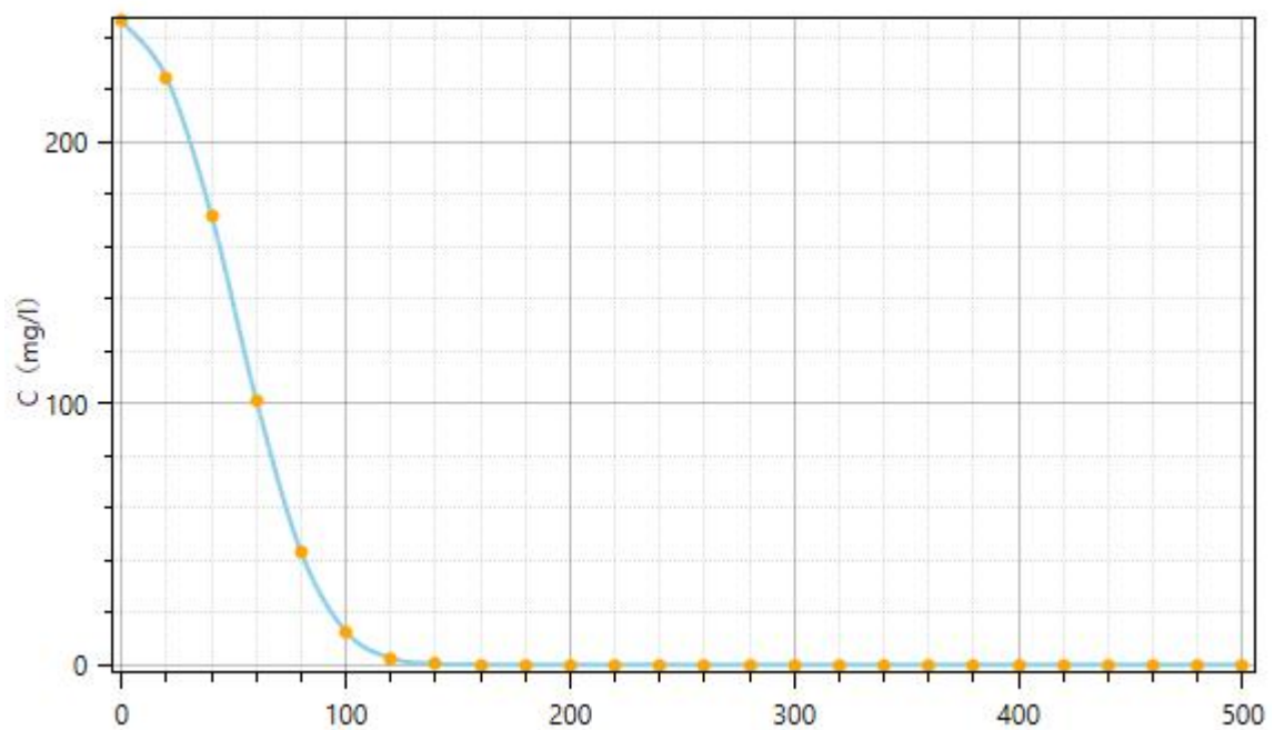
图 4.5-8 废水泄漏 100d 时氨氮影响浓度范围图
