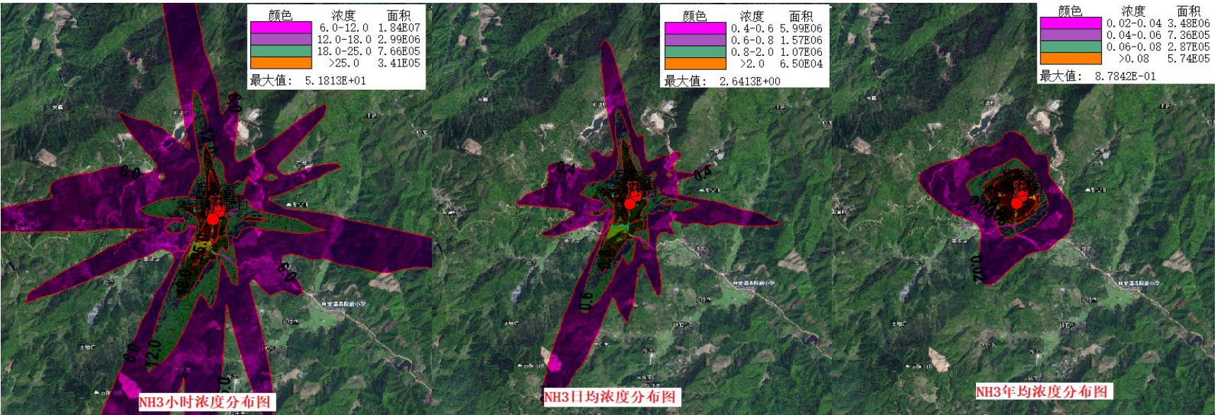
图 4.1-2 \text{NH}_3 排放浓度分布图 (单位: \mu\text{g}/\text{m}^3 )
