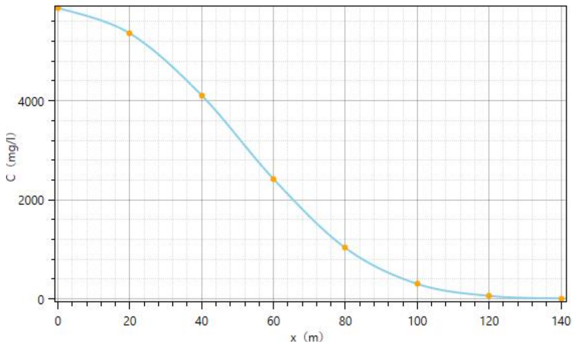
图 4.5-5 废水泄漏 100d 时 COD 影响浓度范围图
