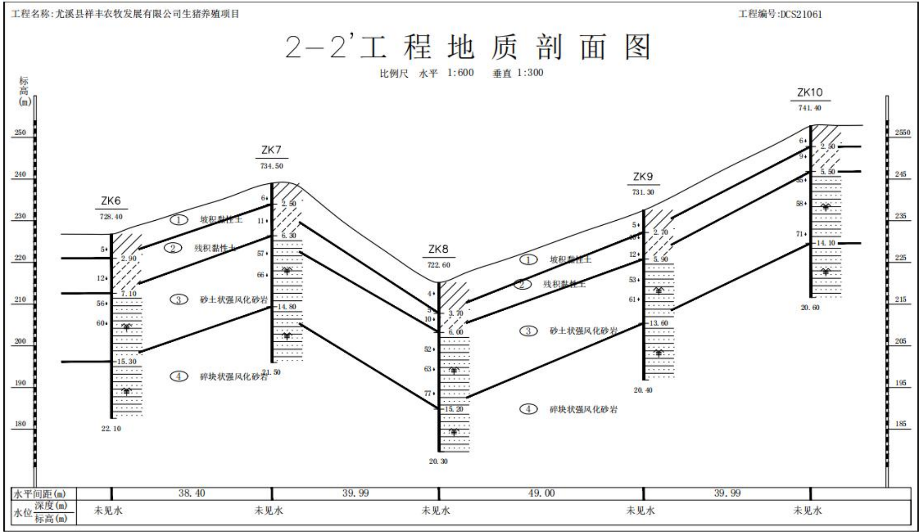
图 4.5-2 工程地质剖面图
