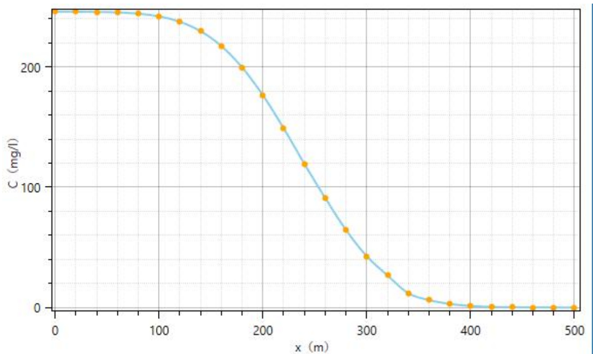
图 4.5-9 废水泄漏 500d 时氨氮影响浓度范围图
