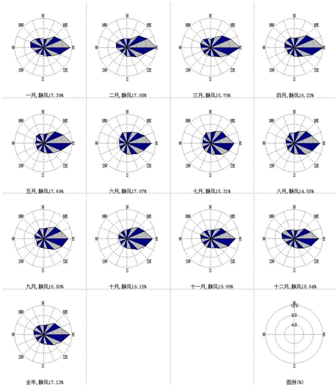
图 4.1-1 尤溪站 2004-2023 年平均风向频率玫瑰图
