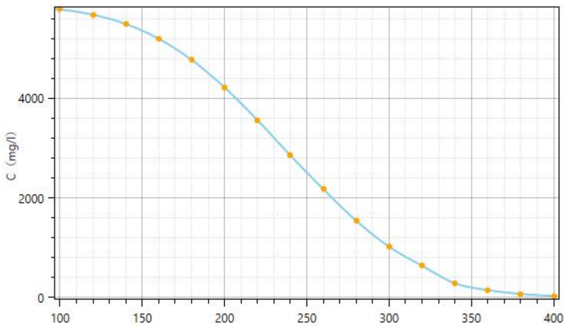
图 4.5-6 废水泄漏 500d 时 COD 影响浓度范围图
