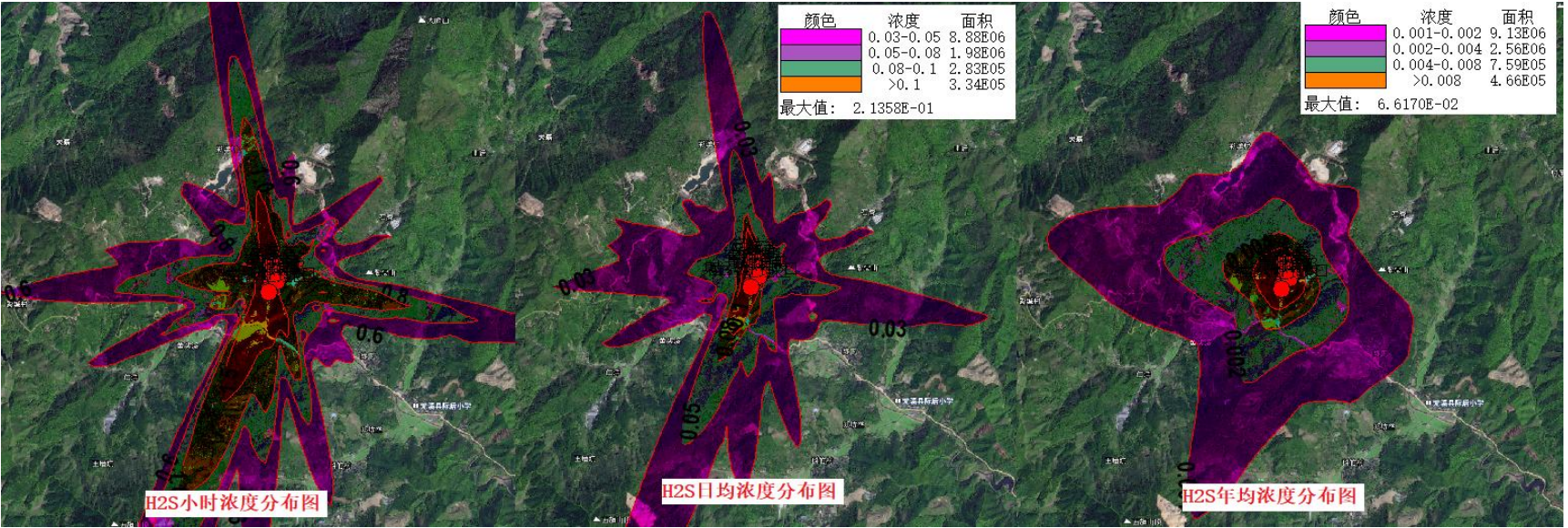
图 4.1-3 \text{H}_2\text{S} 排放浓度分布图 (单位: \mu\text{g}/\text{m}^3 )
