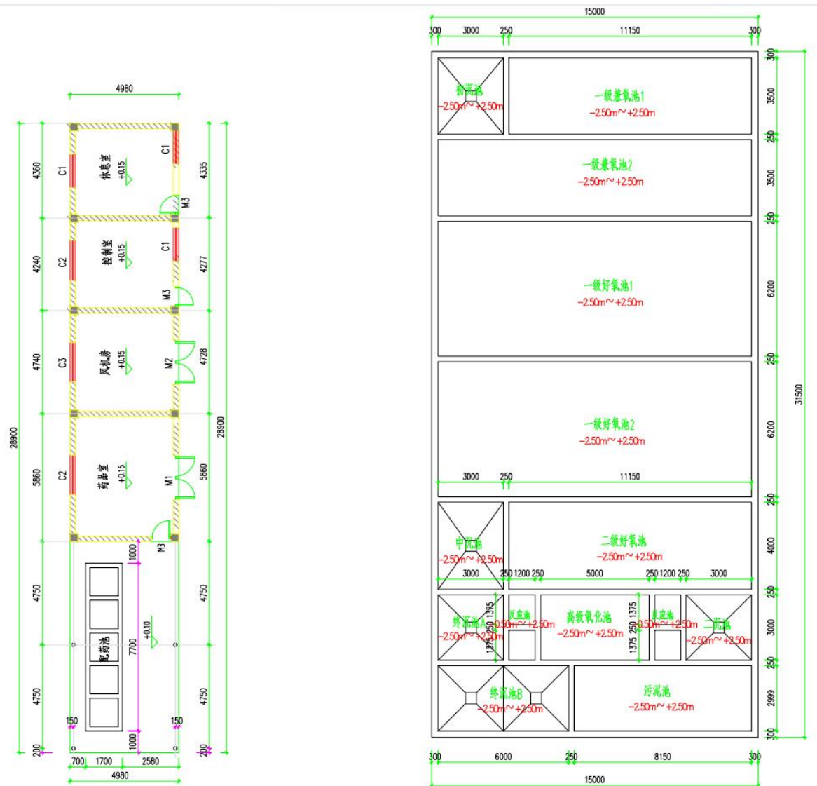
图 2.2-2 污水处理设施平面布置图
