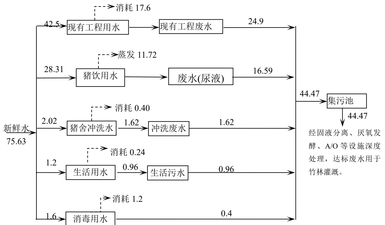
图 2.4-3 冬季全场水平衡图 (单位 t/d)
