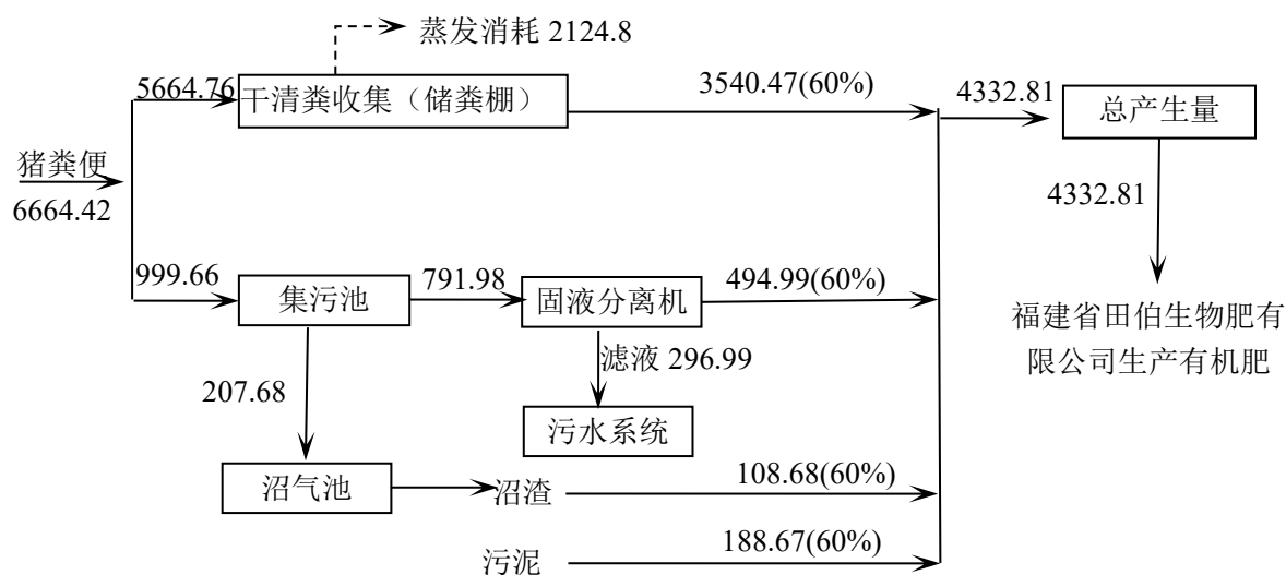
图 2.4-5 扩建后全场粪污平衡图（单位：t/a）
