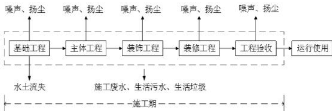
图 2.5-1 施工期工艺流程及产污环节
