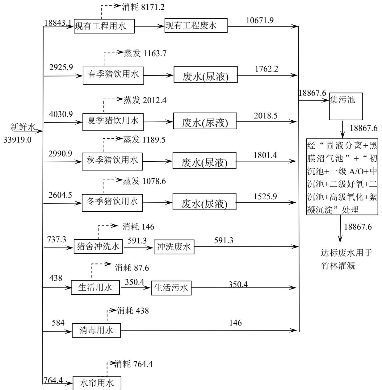
图 2.4-4 项目水平衡图 (单位 t/a)
