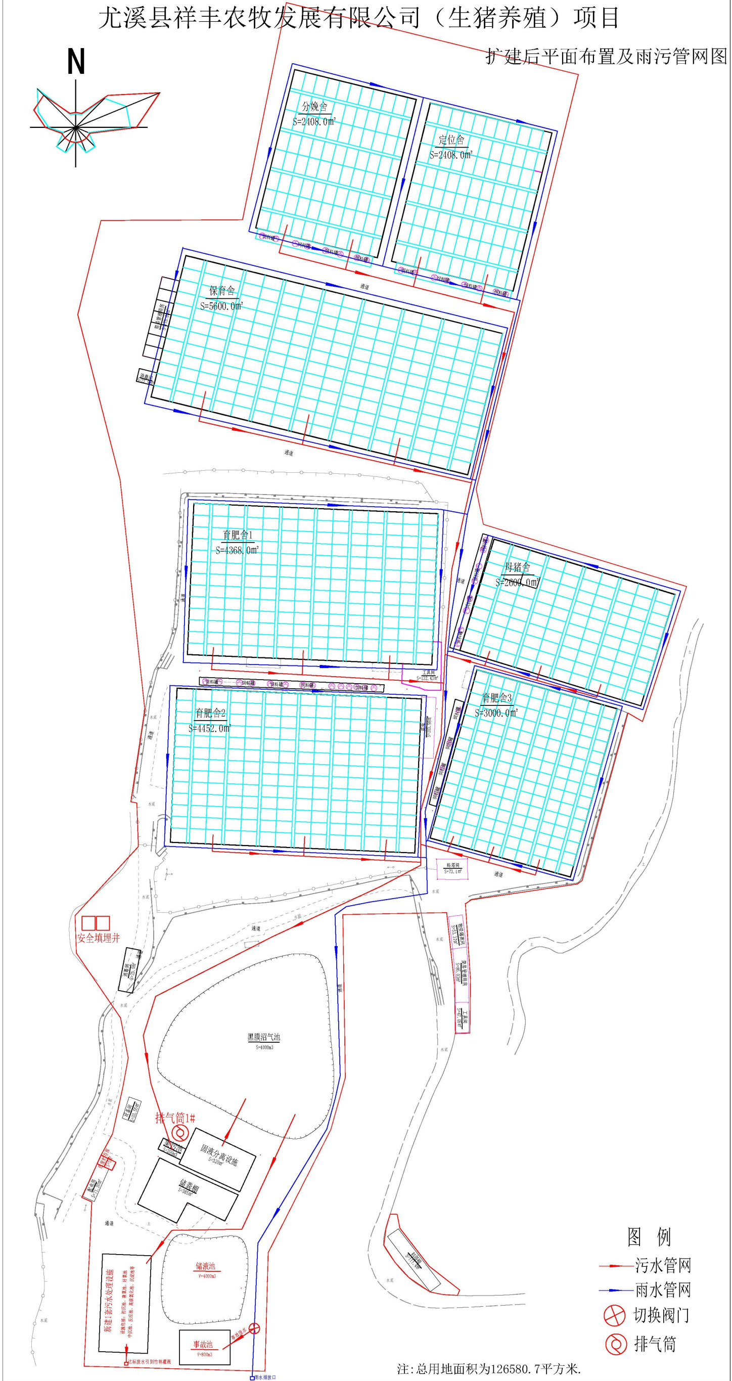
图 2.2-1 养殖场平面布置及雨污管网图
