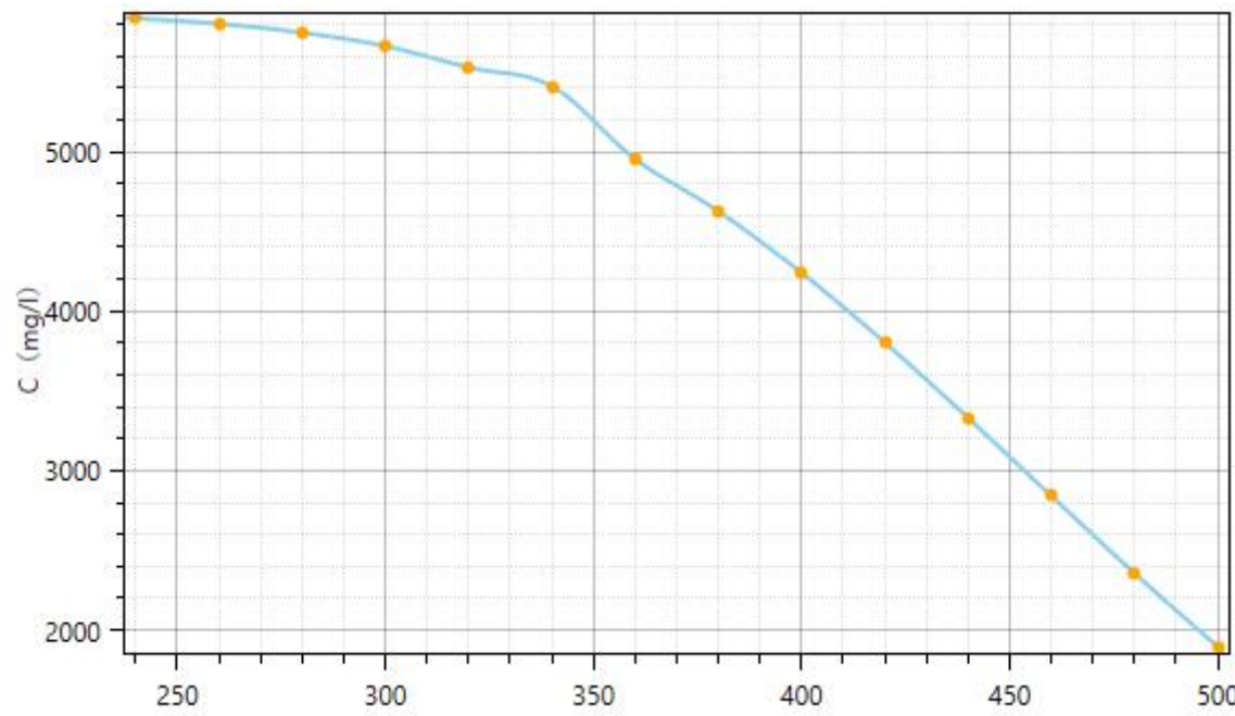
图 4.5-7 废水泄漏 1000d 时 COD 影响浓度范围图
