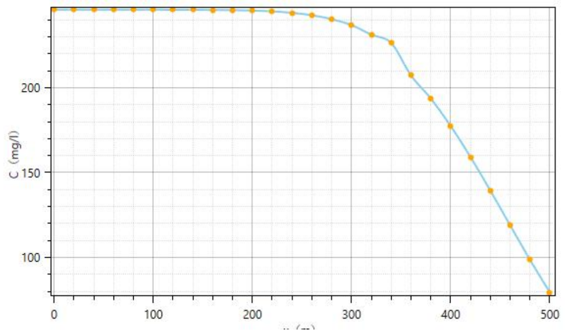
图 4.5-10 废水泄漏 1000d 时氨氮影响浓度范围图
